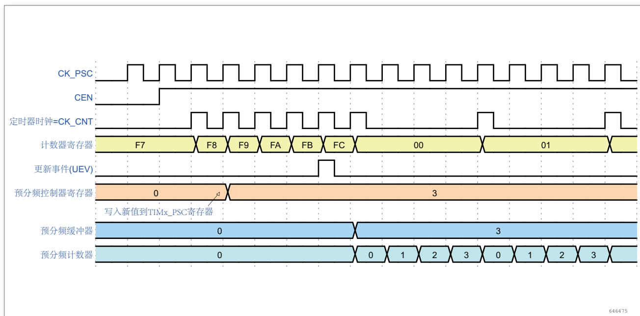
图 38. 当预分频器的参数从 1 变到 4 时，计数器的时序图
