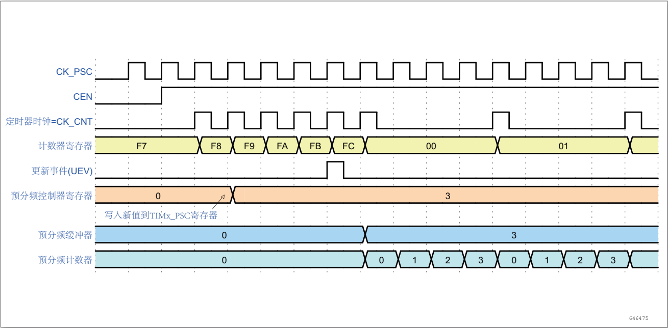
图 86. 当预分频器的参数从 1 变到 4 时，计数器的时序图
