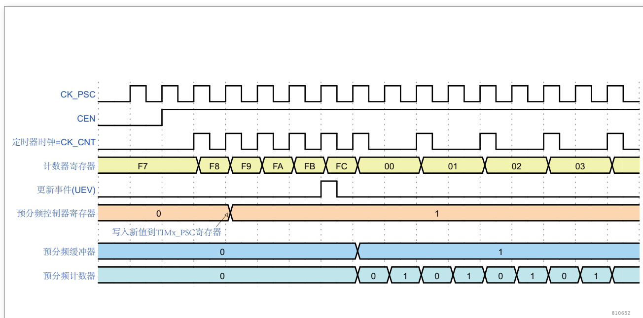
图 37. 当预分频器的参数从 1 变到 2 时，计数器的时序图
