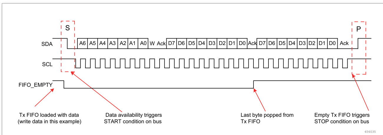
图 163. 主发送 - Tx FIFO 为空
