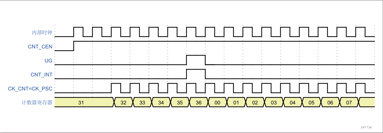
图 104. 一般模式下的控制电路, 内部时钟分频因子为 1
