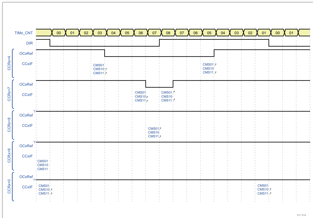
图 69. 中央对齐的 PWM 波形 (APR = 8)
