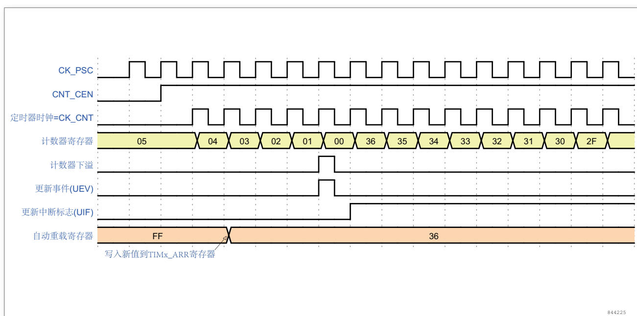
图 97. 计数器时序图，当没有使用重复计数器时的更新事件
