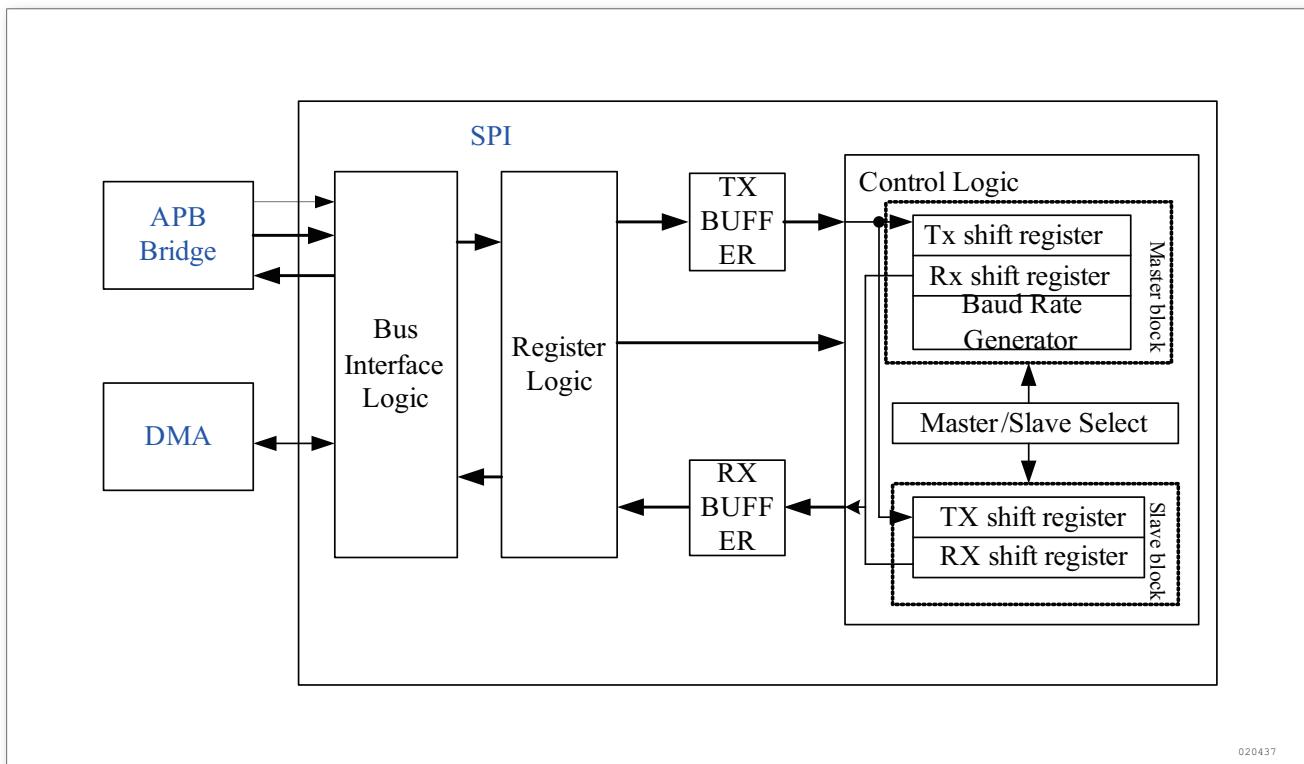
图 153. SPI 框图
