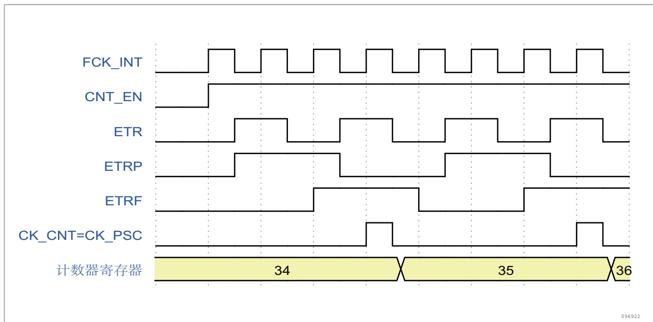
图 61. 外部时钟模式 2 下的控制电路
