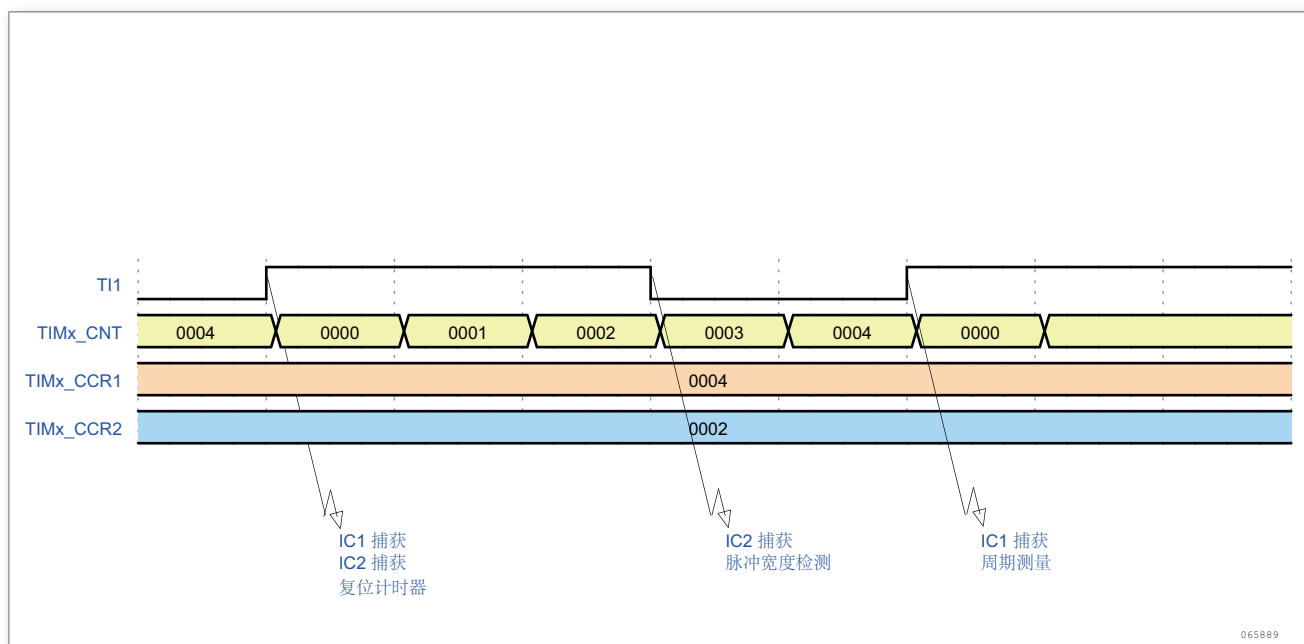
图 66. PWM 输入模式时序
