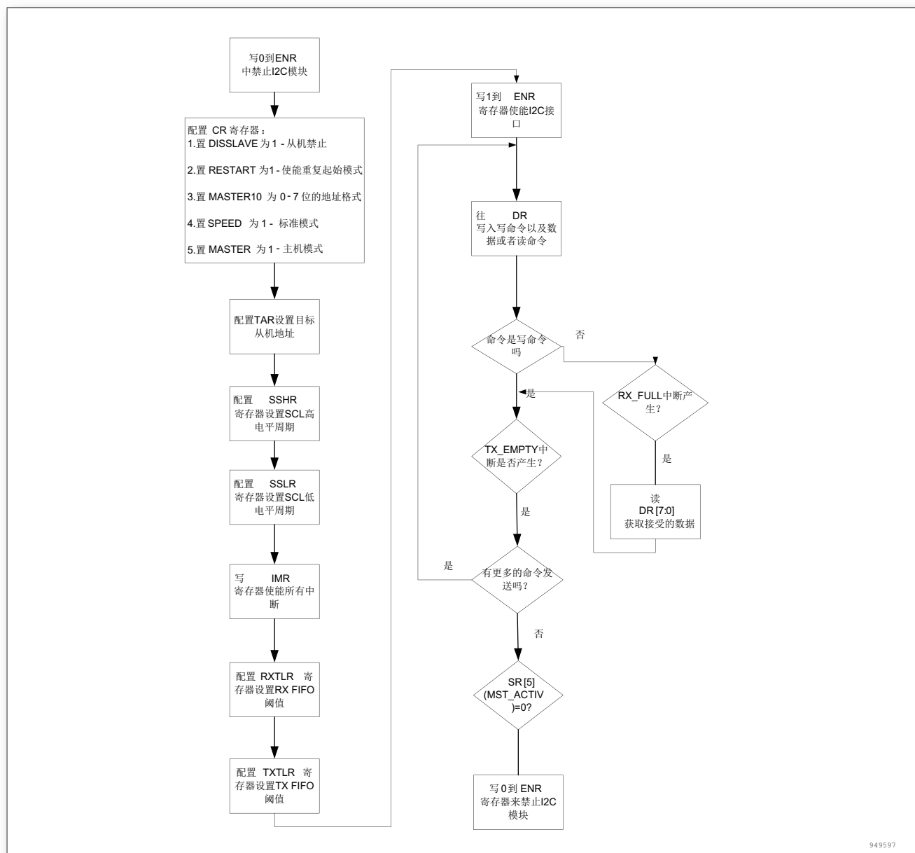
图 168. I2C 接口主机流程图
