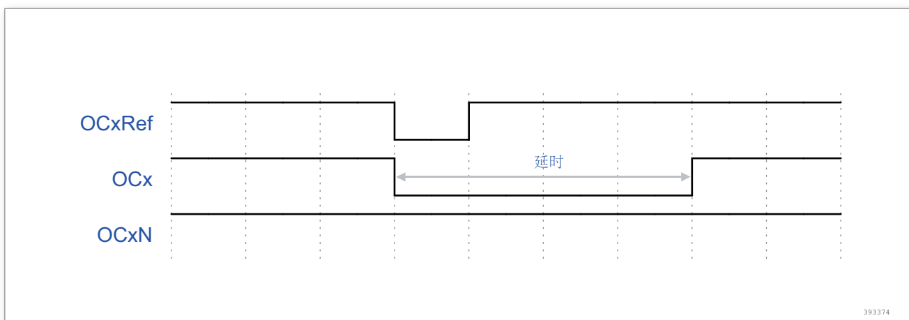
图 71. 死区波形延迟大于负脉冲
