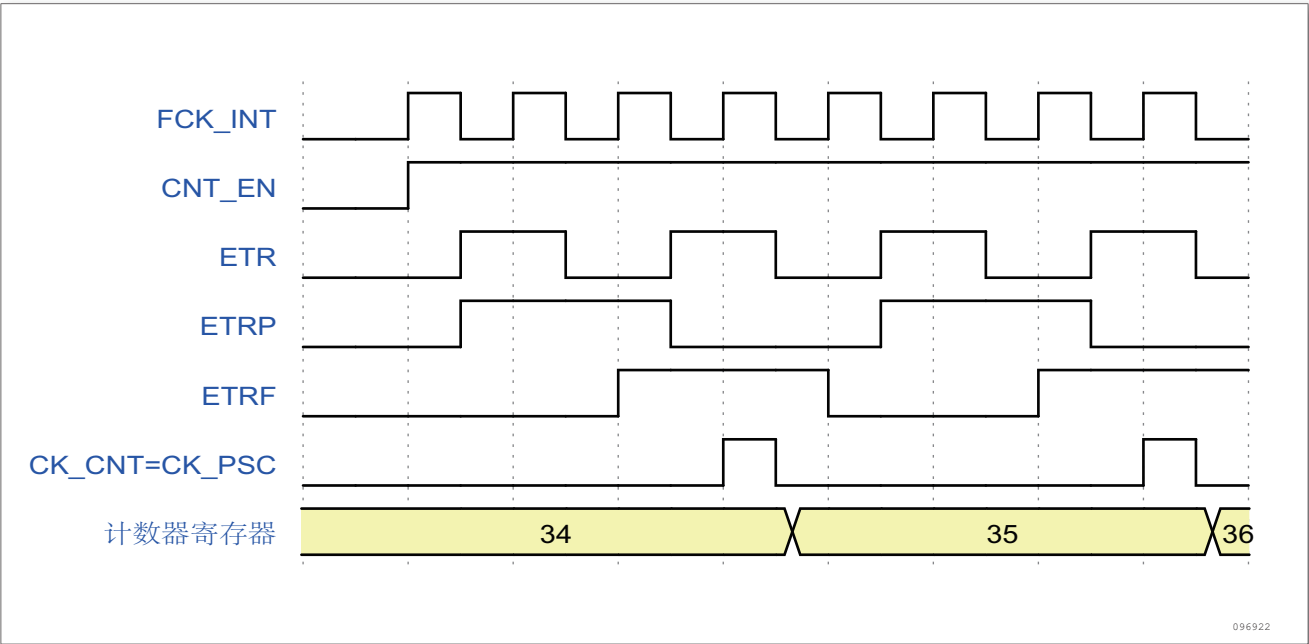
图 108. 外部时钟模式 2 下的控制电路
