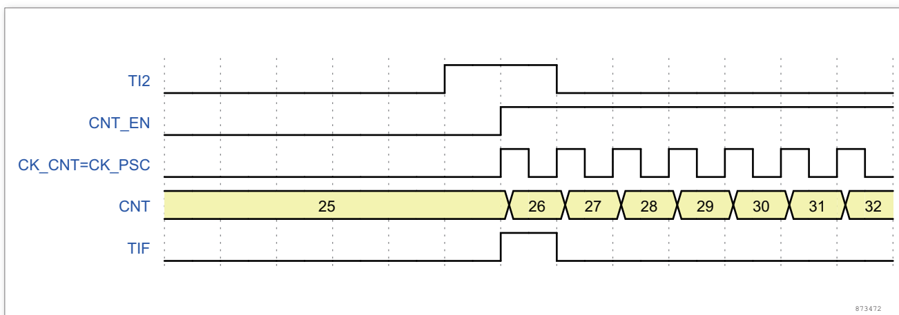
图 82. 触发器模式下的控制电路
