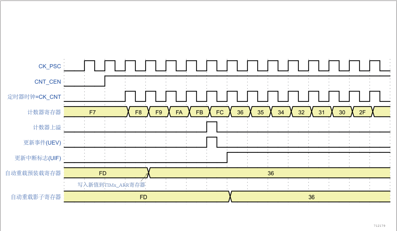
图 103. 计数器时序图，ARPE = 1 时的更新事件 (计数器上溢)
