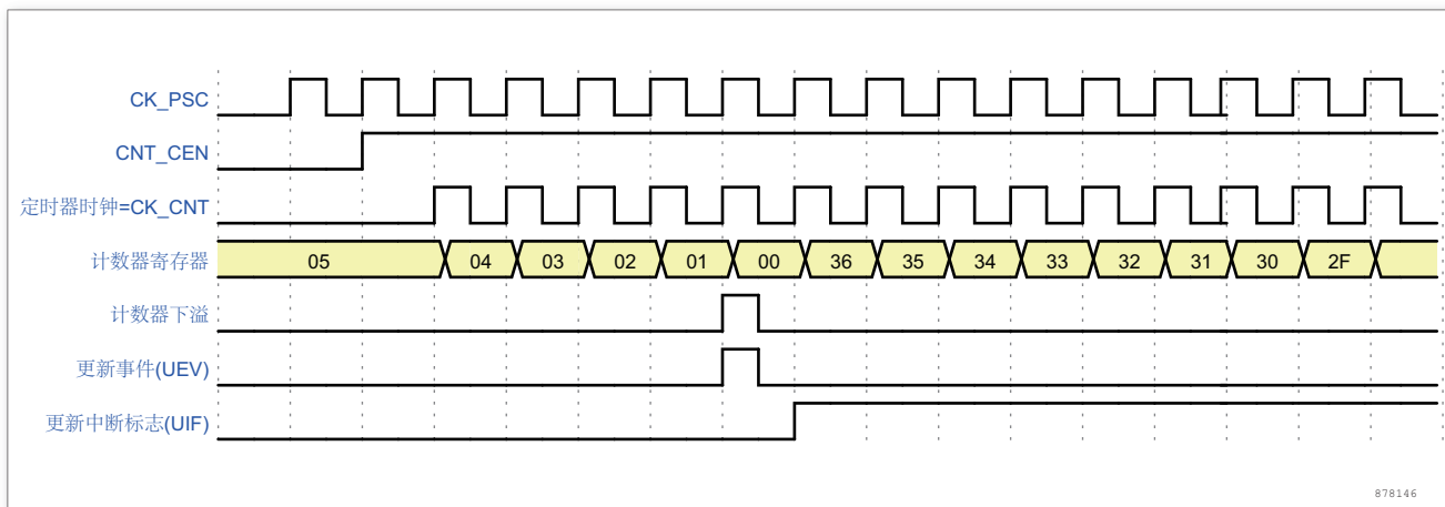
图 45. 计数器时序图，内部时钟分频因子为 1
