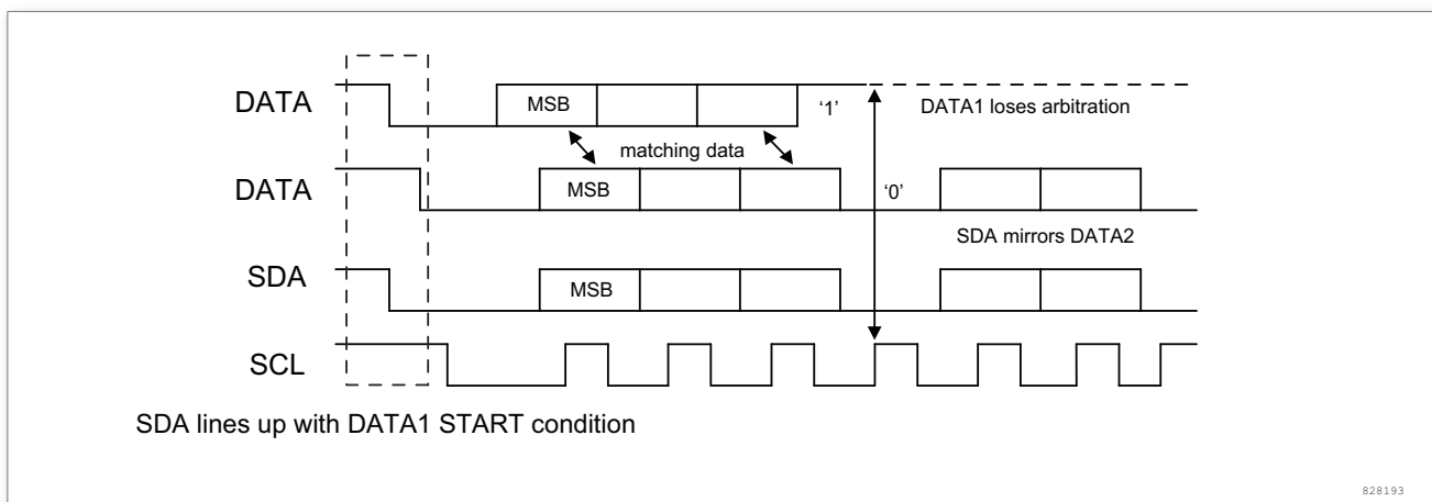
图 165. 多个主机仲裁
