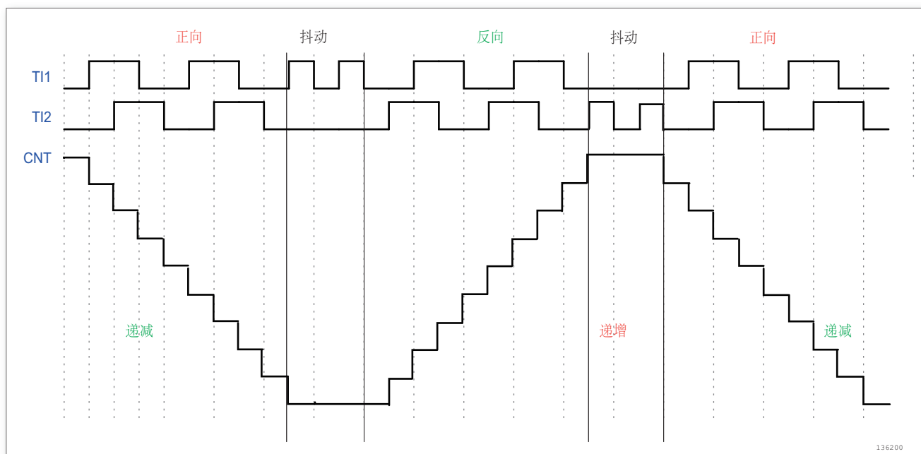
图 78. IC1FP1 反相的编码器接口模式实例
