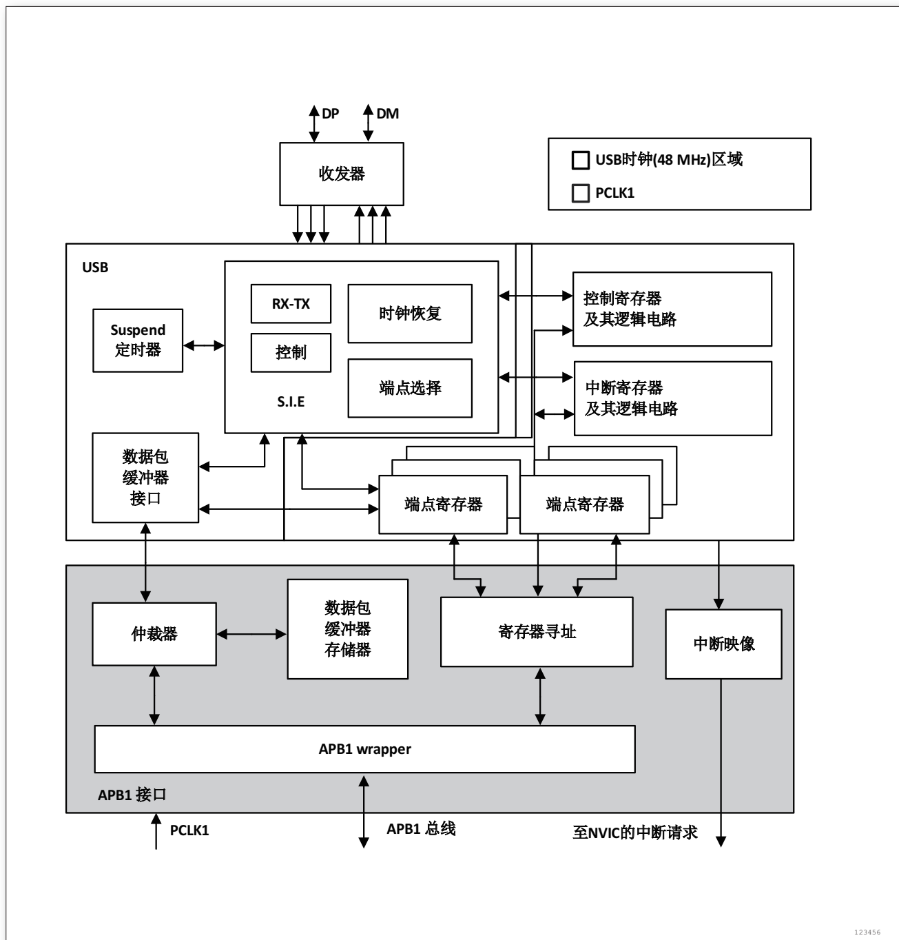
图 136. USB 方框图
