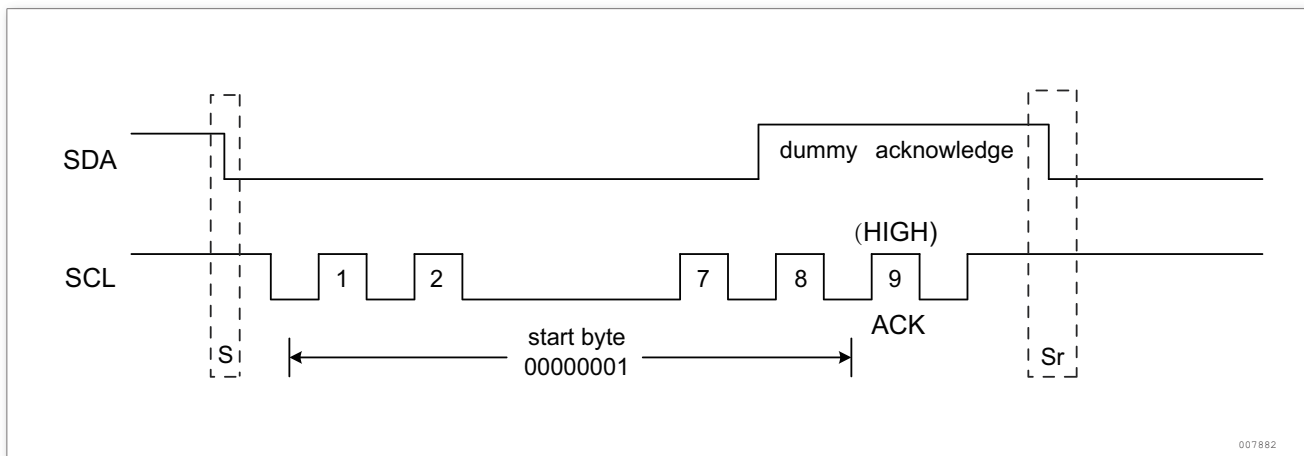
图 161. 起始字节传输
