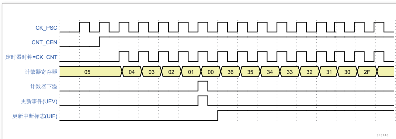
图 93. 计数器时序图，内部时钟分频因子为 1
