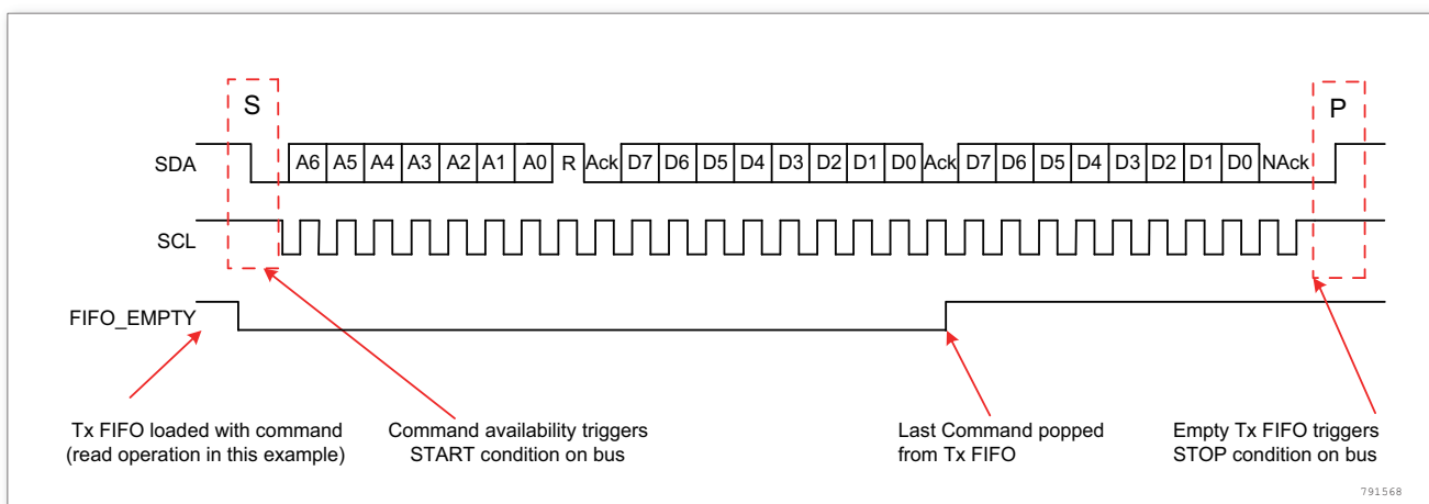
图 164. 主接收 - Tx FIFO 为空
