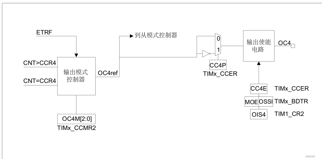
图 65. 捕获/比较通道的输出部分 (通道 4)
