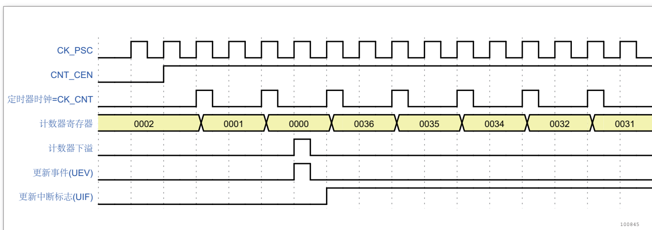
图 46. 计数器时序图，内部时钟分频因子为 2
