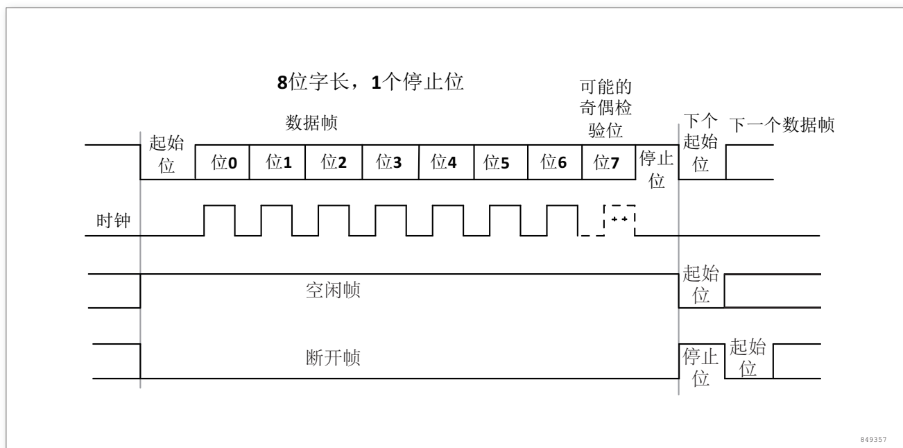
图 171. UART 时序
