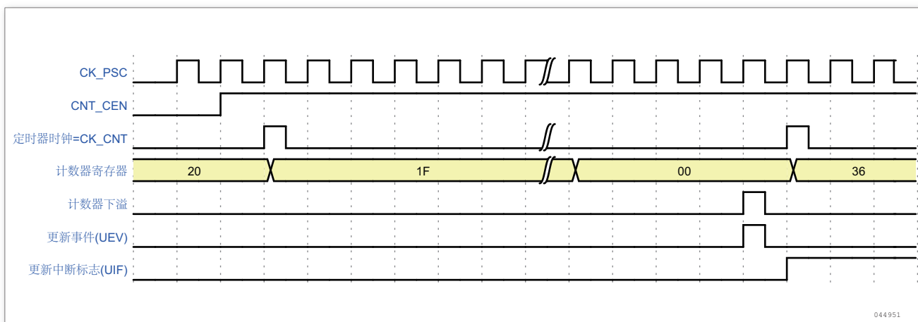
图 96. 计数器时序图，内部时钟分频因子为 N
