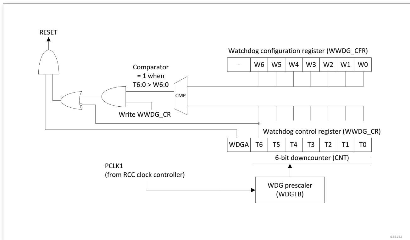
图 134. 看门狗框图
