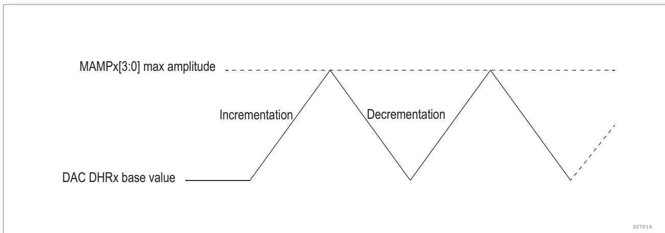
图 34. DAC 三角波生成
