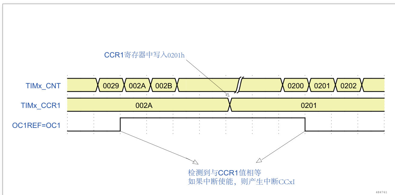
图 113. 输出比较模式, 翻转 OC1
