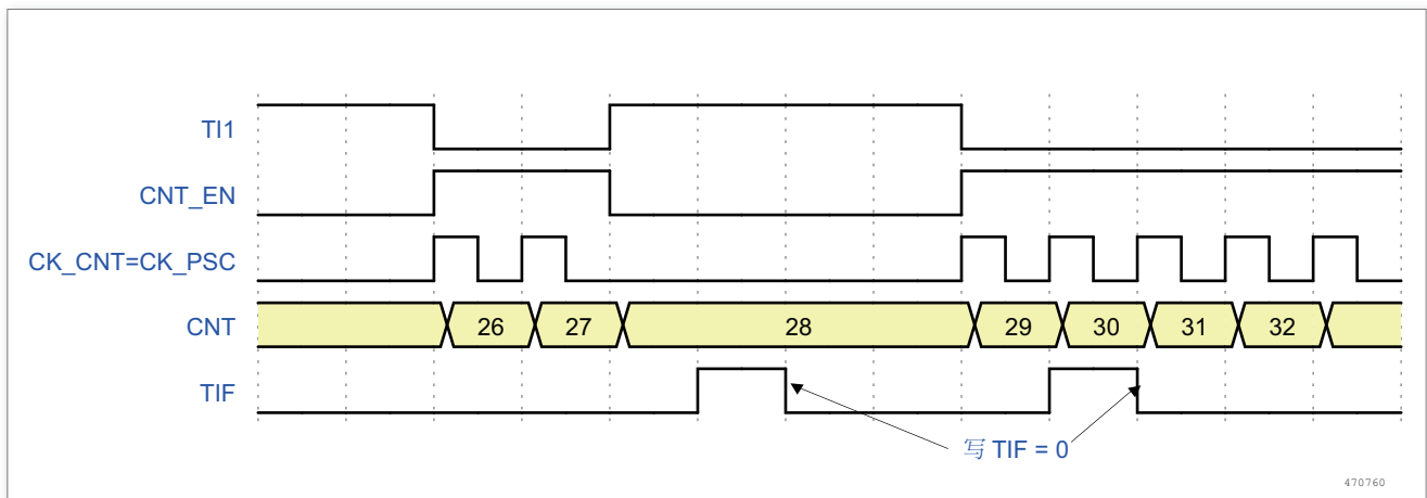
图 121. 门控模式下的控制电路
