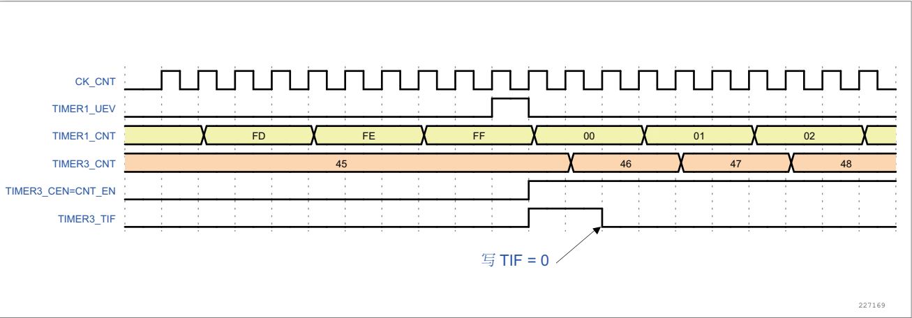
图 127. 使用定时器 1 的更新触发定时器 2
