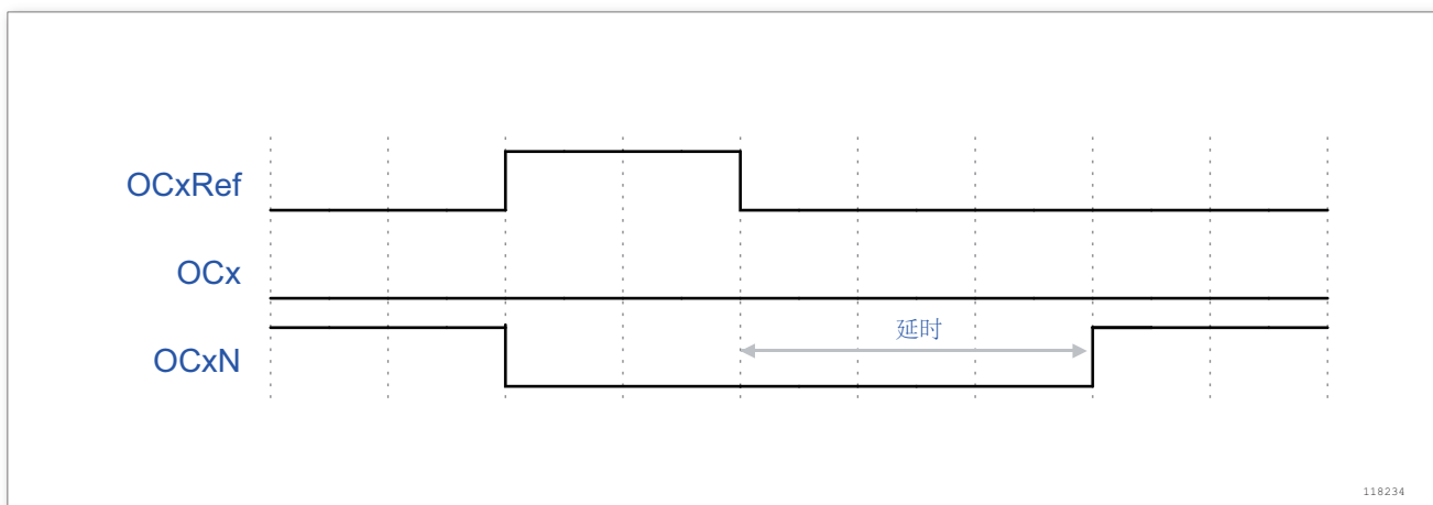
图 72. 死区波形延迟大于正脉冲
