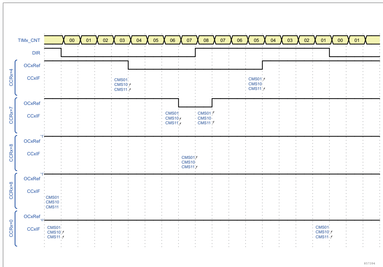
图 115. 中央对齐的 PWM 波形 (APR = 8)
