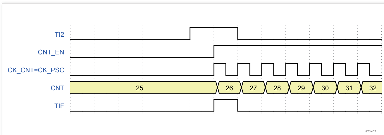
图 122. 触发器模式下的控制电路
