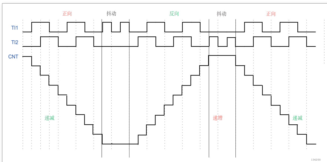
图 119. IC1FP1 反相的编码器接口模式实例
