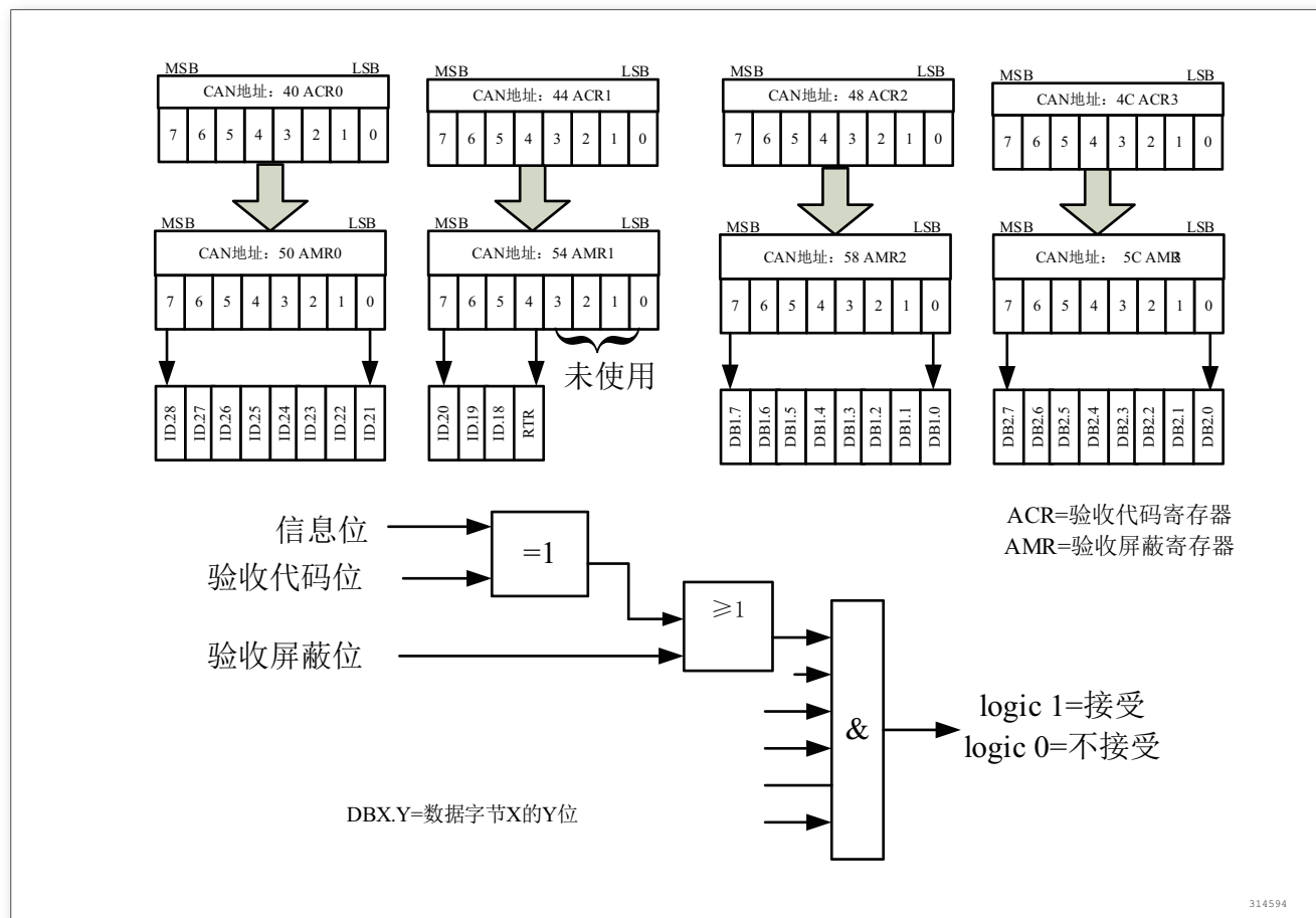
图 145. 接收标准结构信息时的单个滤波器配置
