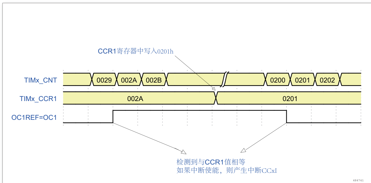
图 67. 输出比较模式，翻转 OC1
