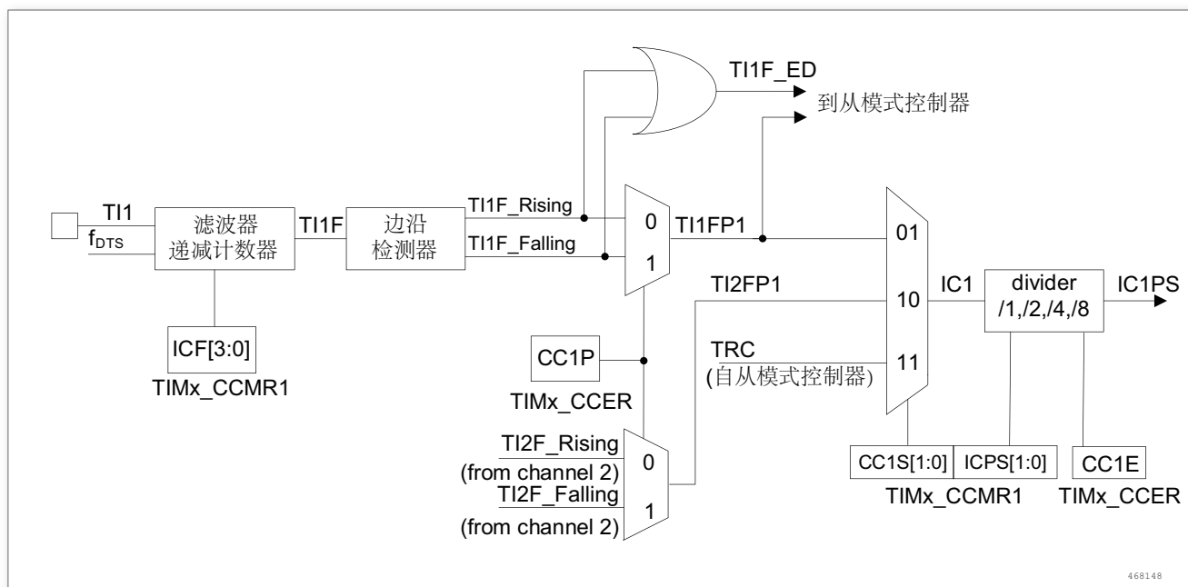
图 62. 捕获/比较通道 (如：通道 1 输入部分)
