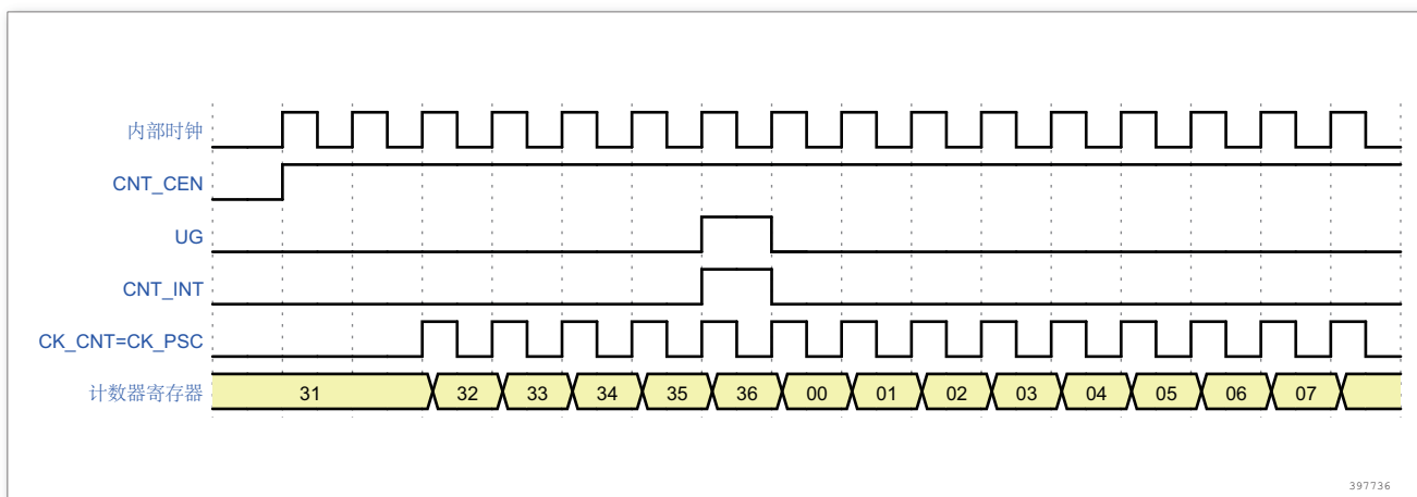
图 57. 一般模式下的控制电路，内部时钟分频因子为 1
