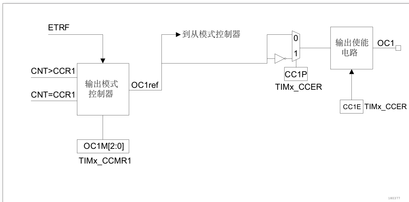
图 64. 捕获/比较通道的输出部分 (通道 1 至 3)
