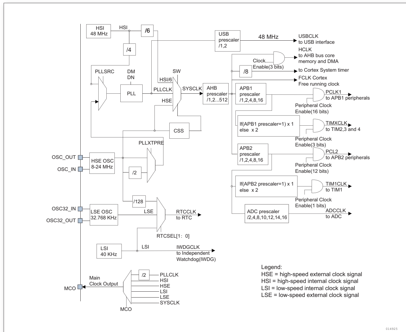
图 12. 时钟树
