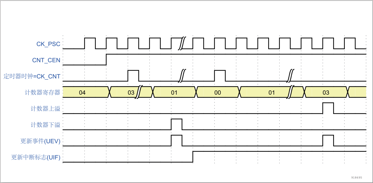
图 101. 计数器时序图，内部时钟分频因子为 N
