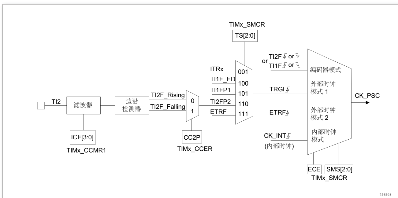
图 58. TI2 外部时钟连接例子
