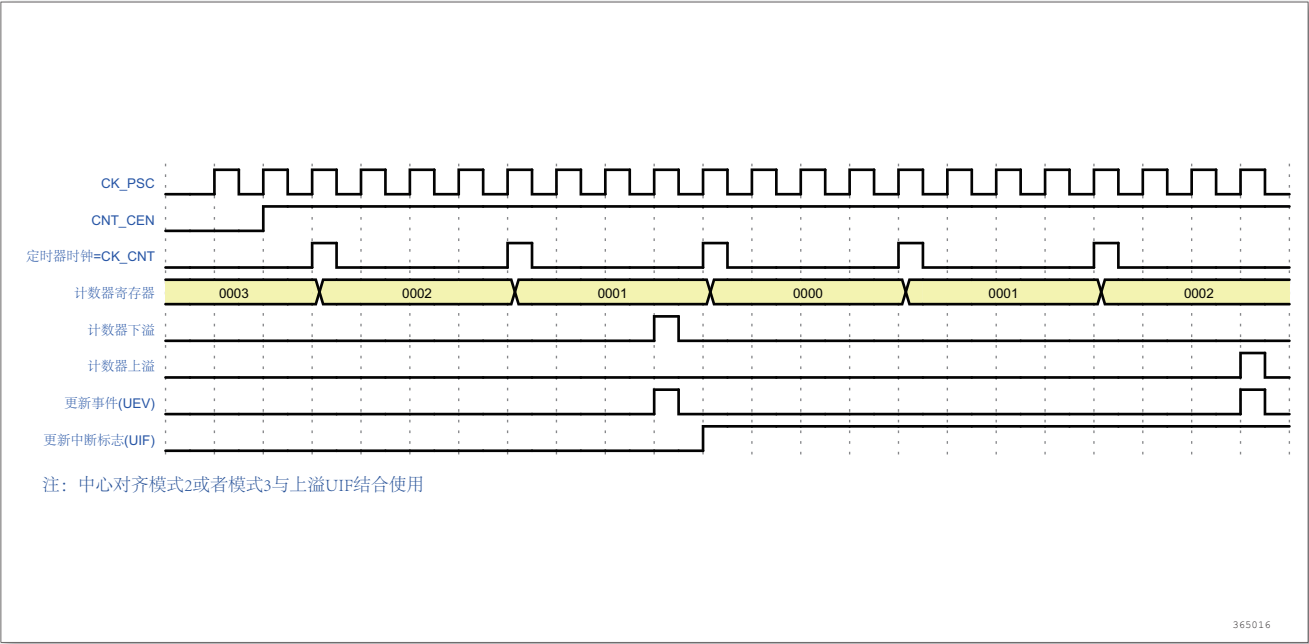
图 52. 计数器时序图，内部时钟分频因子为 4，TIMx_ARR = 0x03
