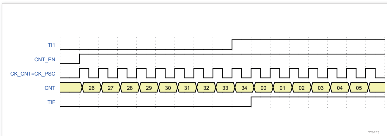
图 80. 复位模式下的控制电路
