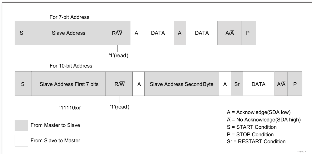
图 160. 主接收协议
