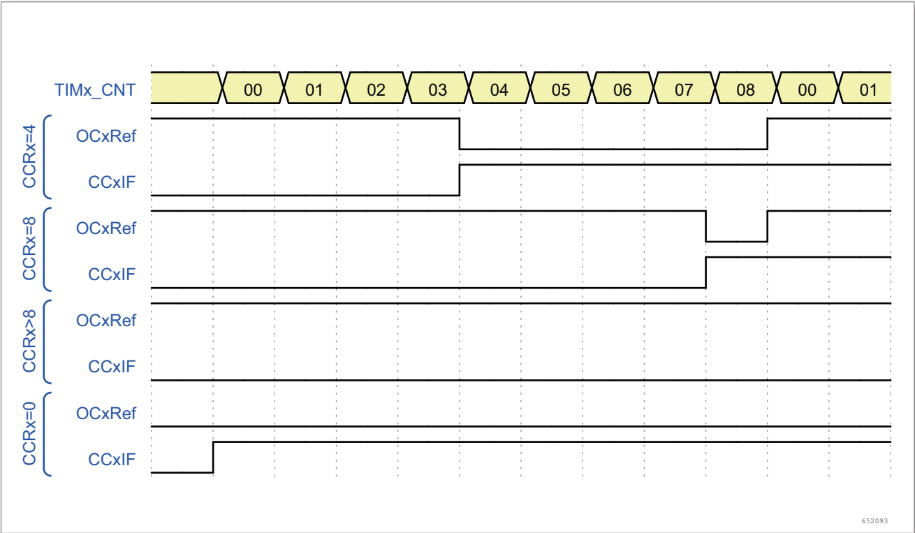
图 114. 边沿对齐的 PWM 波形 (ARR = 8)
