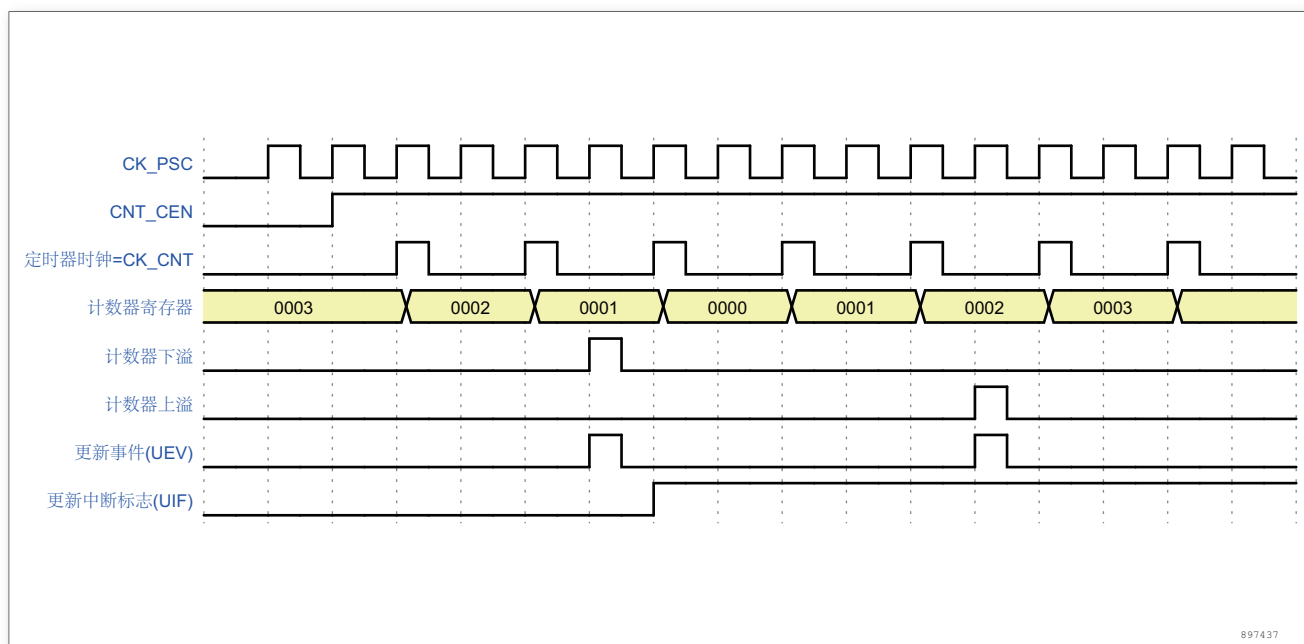
图 99. 计数器时序图，内部时钟分频因子为 2
