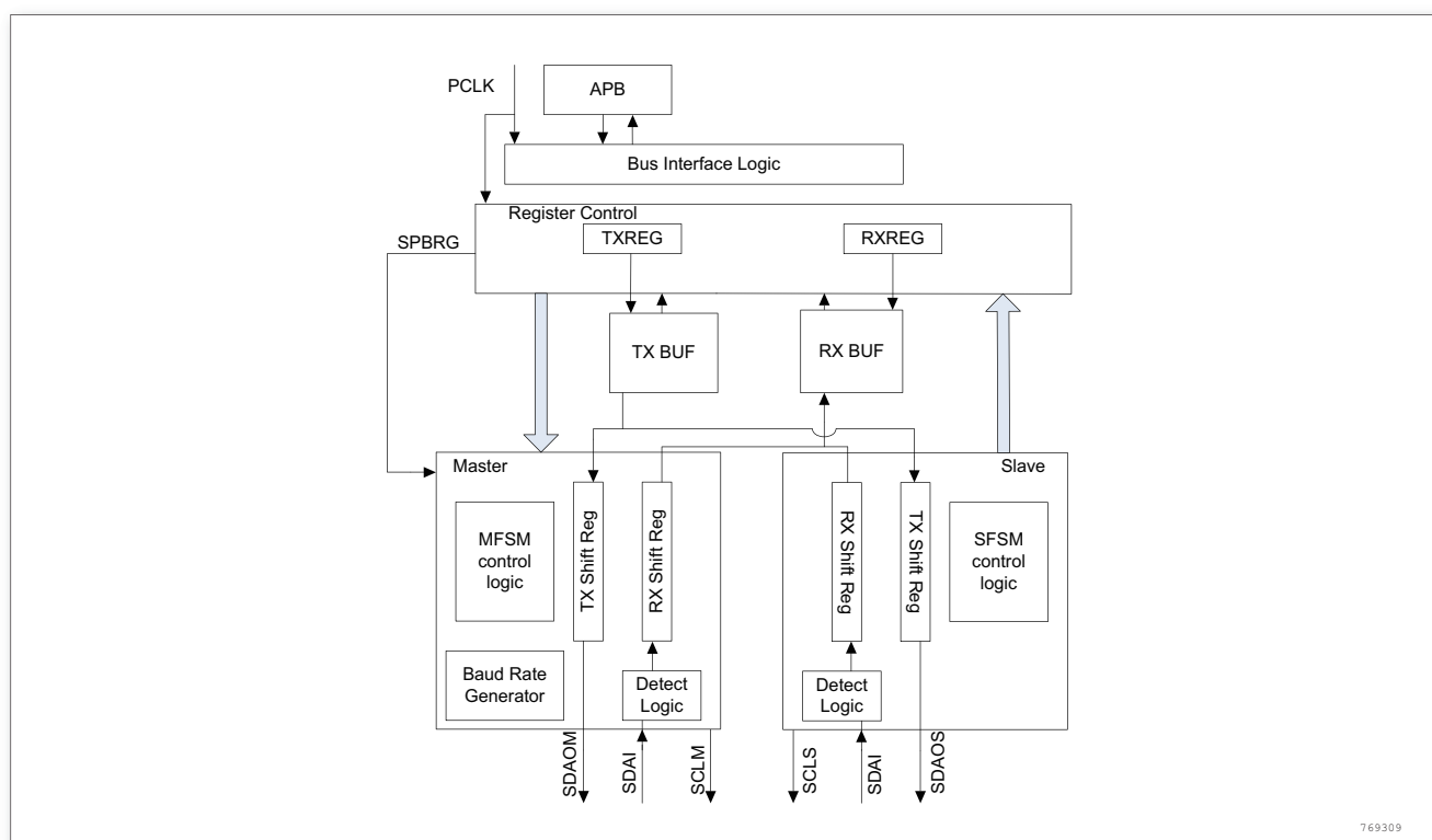
图 167. I2C 功能框图
