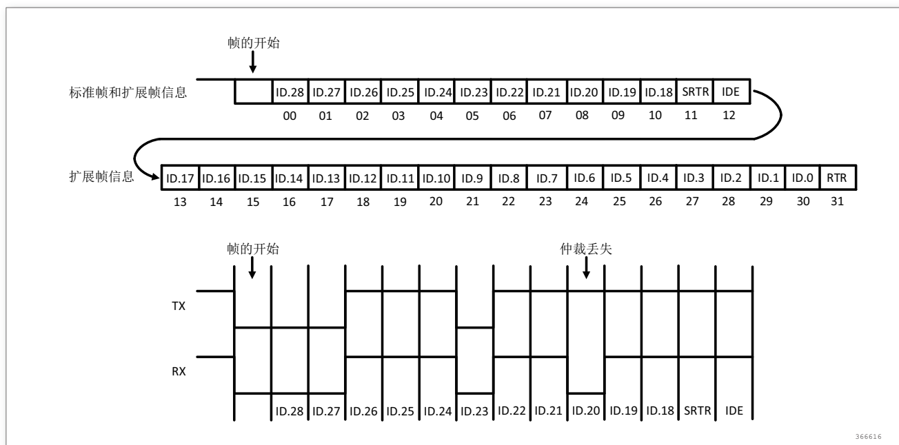
图 152. 仲裁丢失解释举例
