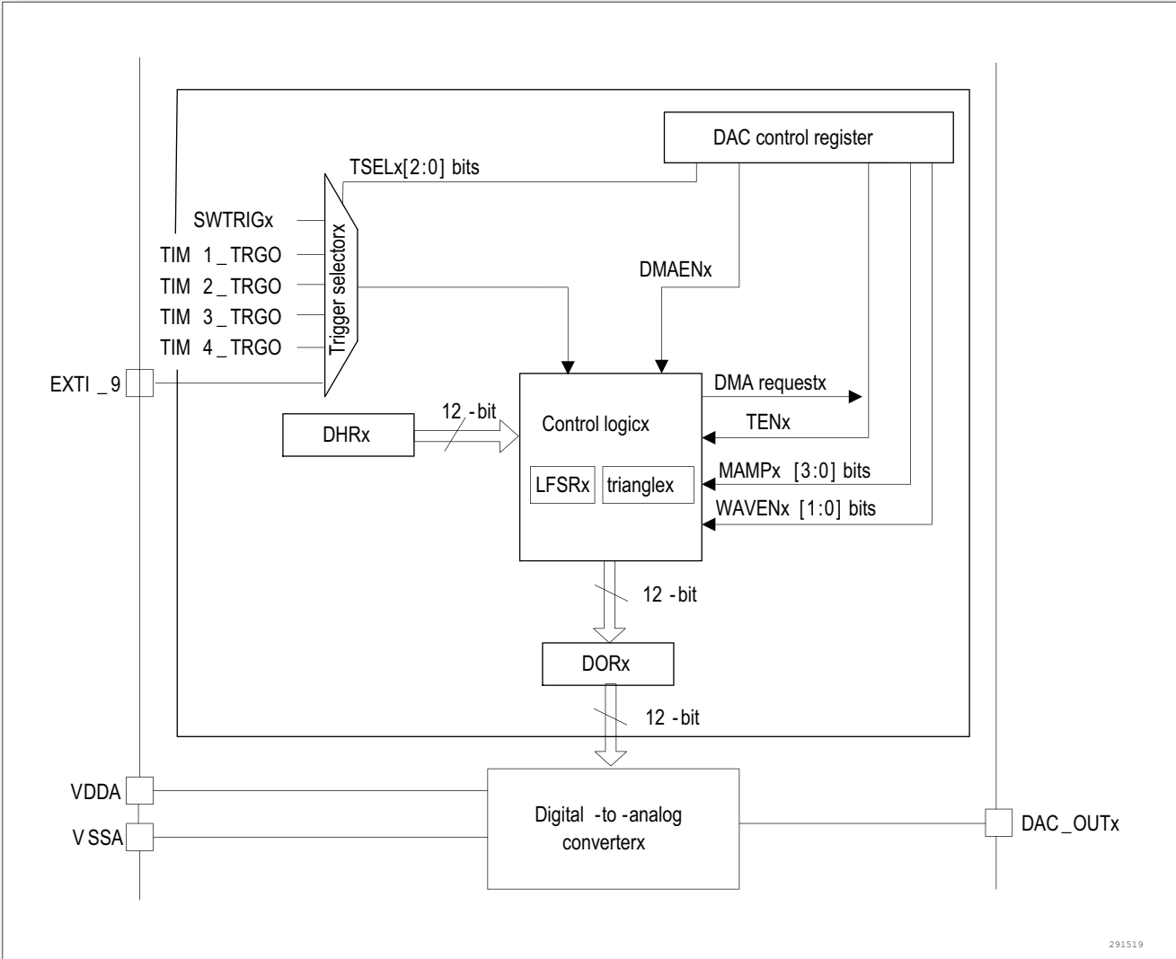
图 28. DAC 通道模块框图
