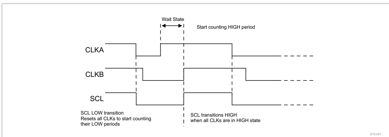
图 166. 多个主机时钟同步
