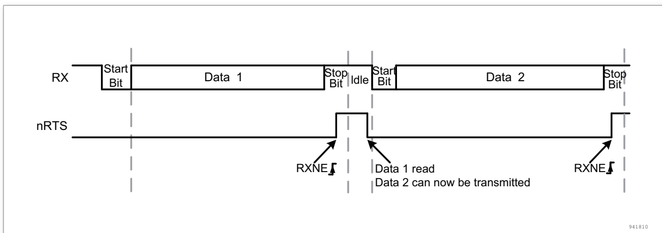
图 177. RTS 流控制
