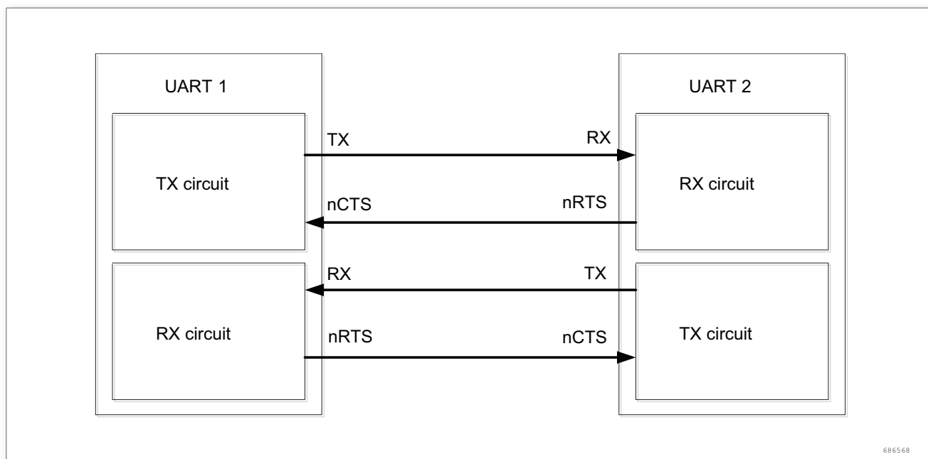
图 176. 两个 UART 间的硬件流控制
