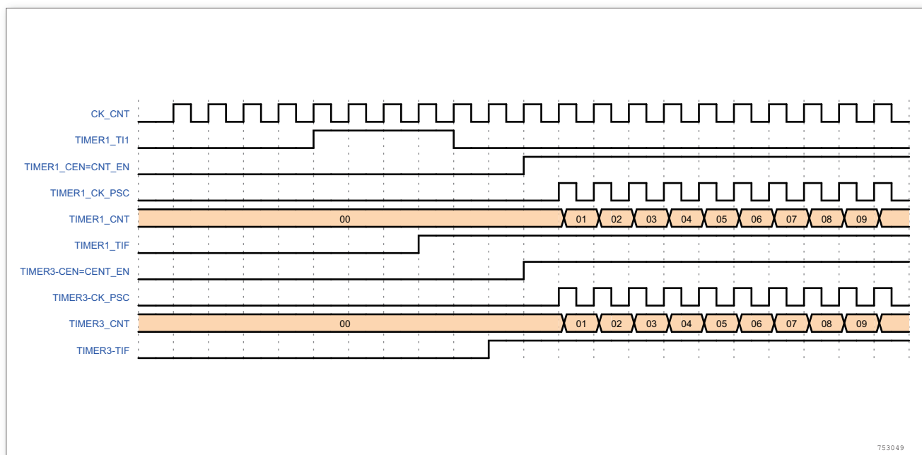
图 129. 使用定时器 1 的 TI1 输入触发定时器 1 和定时器 2
