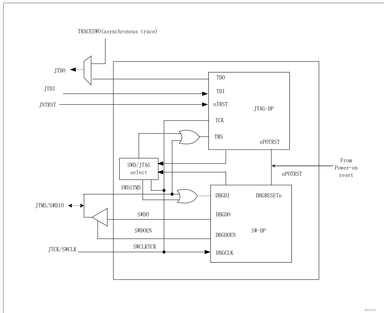
图 180. SWJ 调试端口
