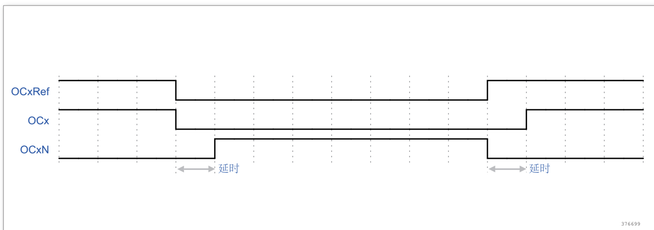
图 70. 带死区插入的互补输出
