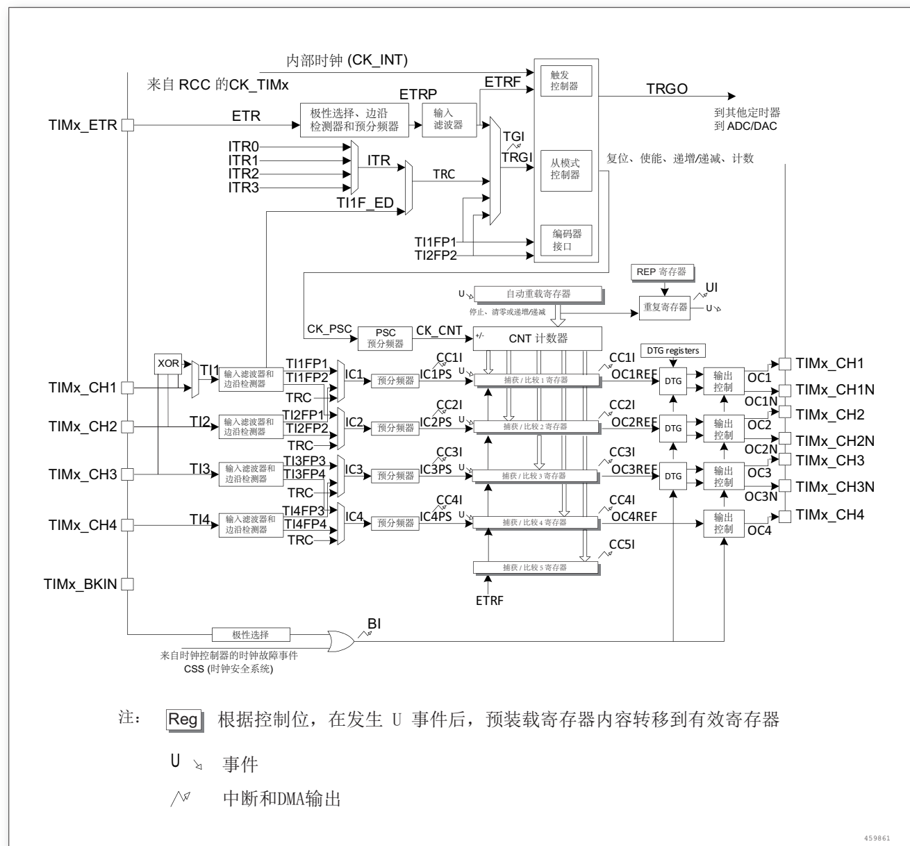
图 36. 高级控制定时器框图
