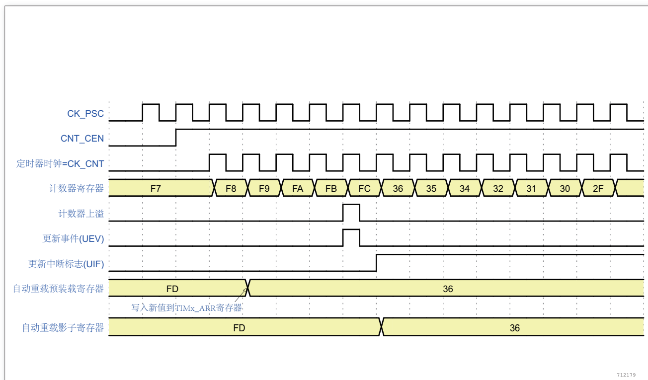
图 55. 计数器时序图, ARPE = 1 时的更新事件 (计数器上溢)
