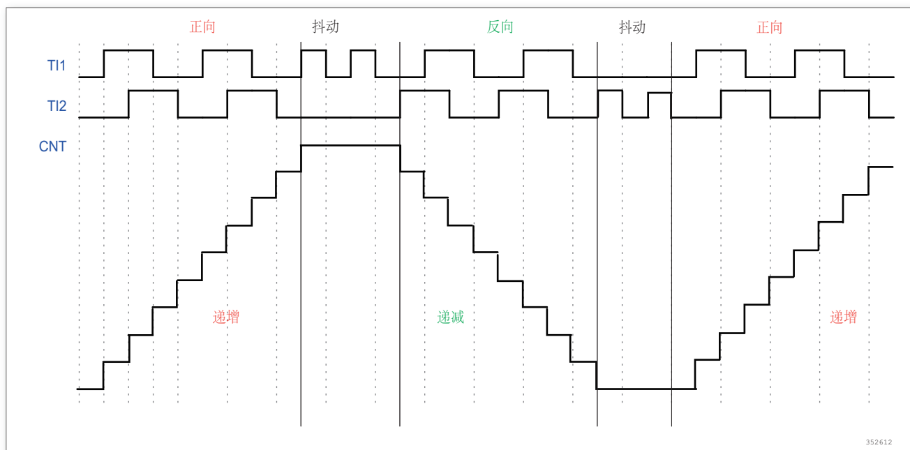
图 77. 编码器模式下的计数器操作实例
