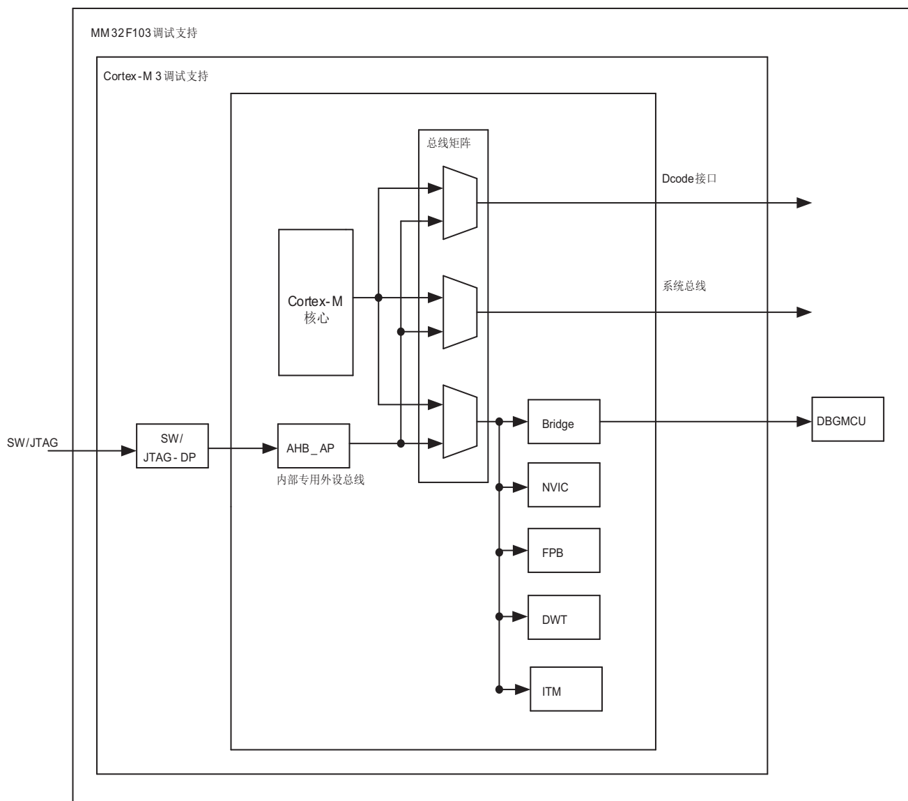
图 179. MM32 系列级别和 CPU 级别的调试框
