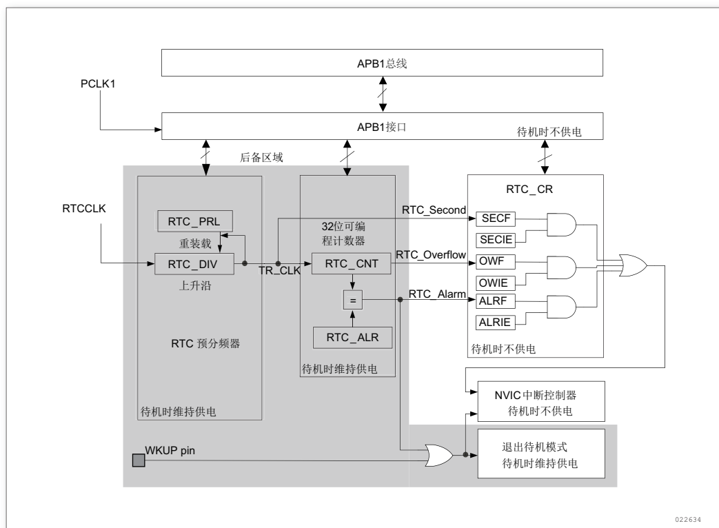
图 130. 实时时钟方框图
