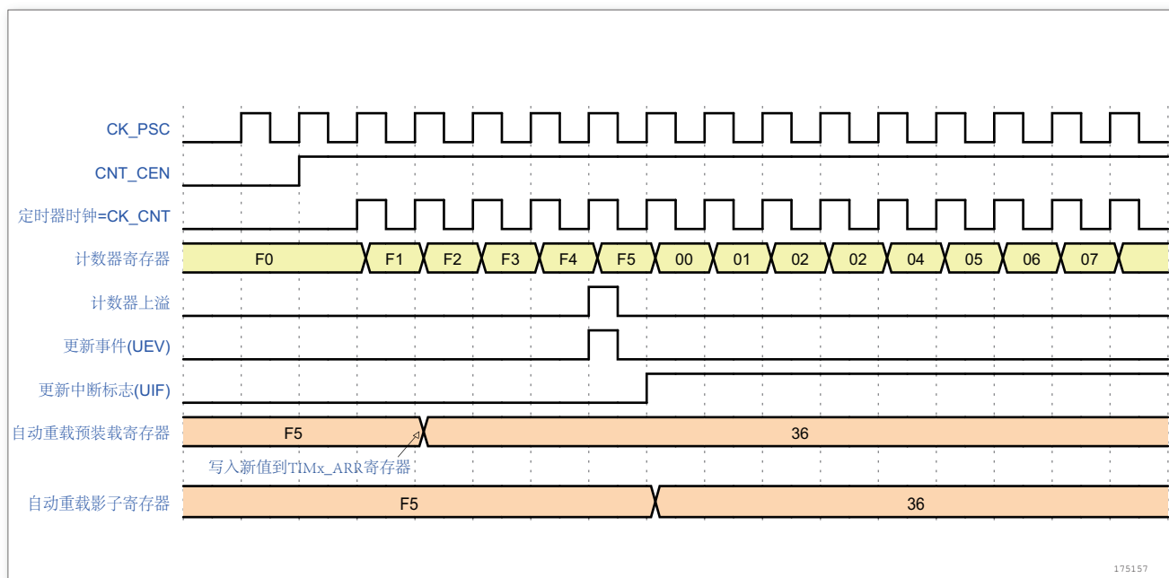
图 92. 计数器时序图，当 ARPE = 1 时的更新事件 (预装入了 TIMx_ARR)
