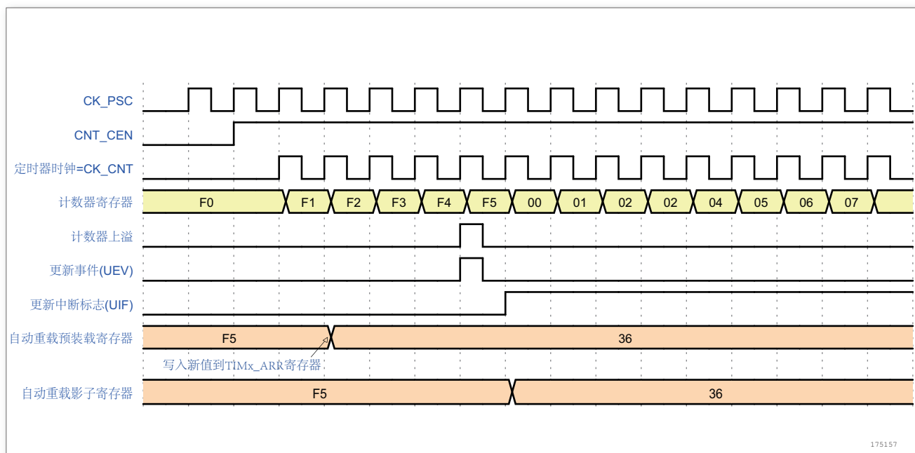
图 44. 计数器时序图，当 ARPE = 1 时的更新事件 (预装入了 TIMx_ARR)
