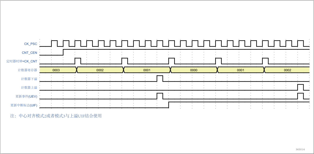
图 100. 计数器时序图，内部时钟分频因子为 4，TIMx_ARR = 0x03
