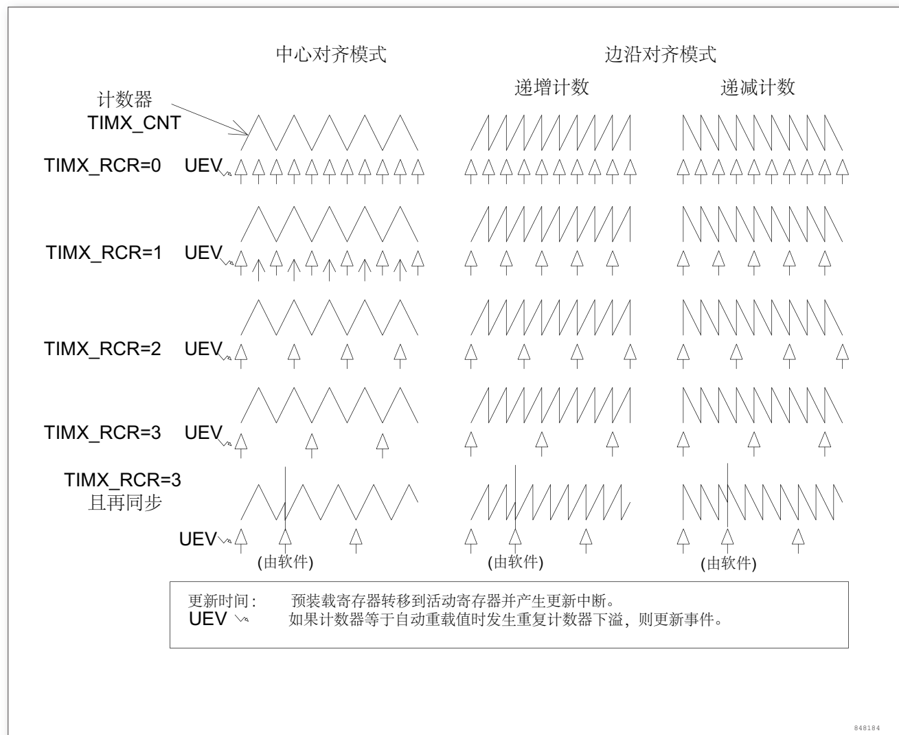
图 56. 不同模式下更新速率的例子, 及 TIMx_RCR 的寄存器设置
