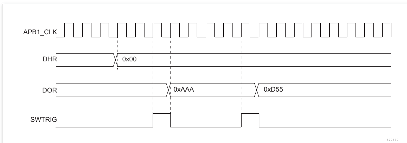
图 33. 带 LFSR 波形生成的 DAC 转换 (使能软件触发)
