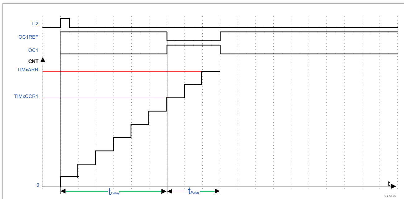
图 116. 单脉冲模式的例子
