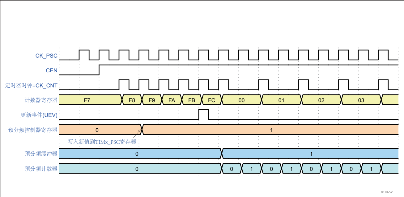
图 85. 当预分频器的参数从 1 变到 2 时，计数器的时序图
