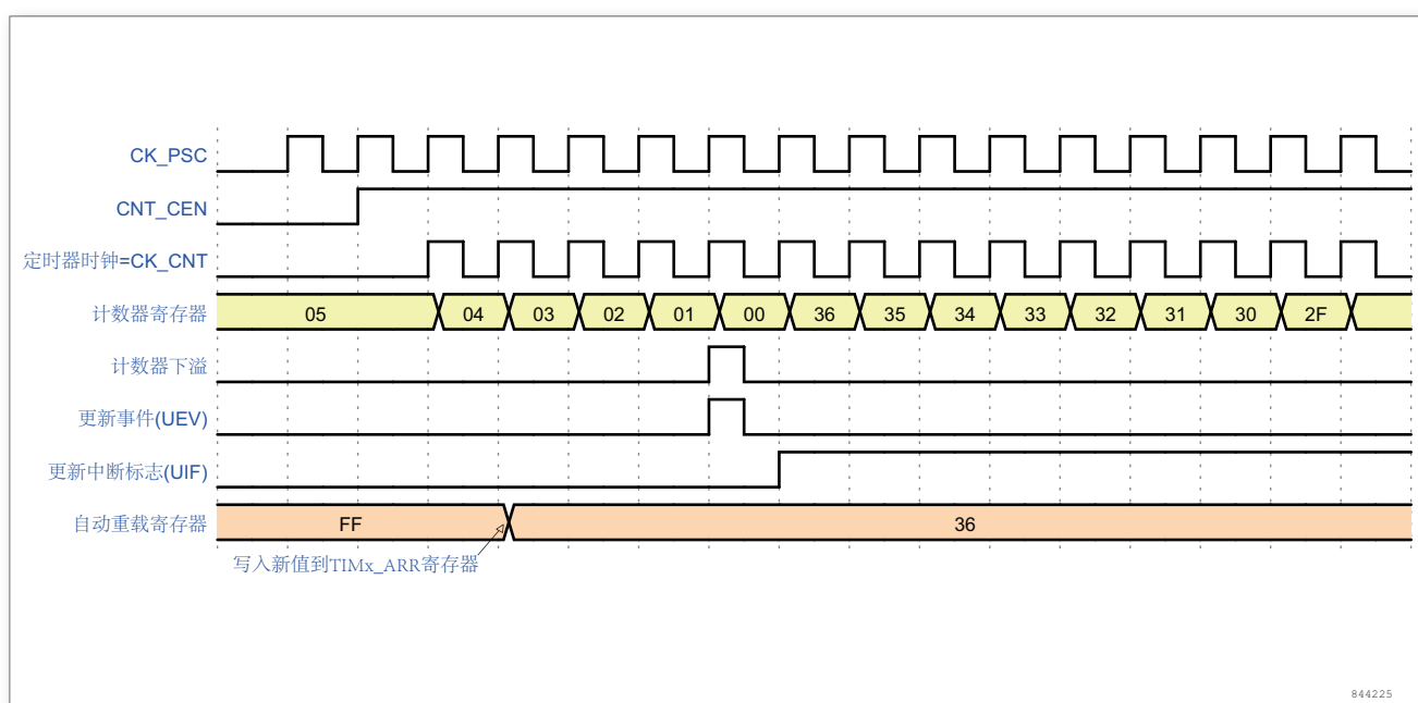
图 49. 计数器时序图, 当没有使用重复计数器时的更新事件
