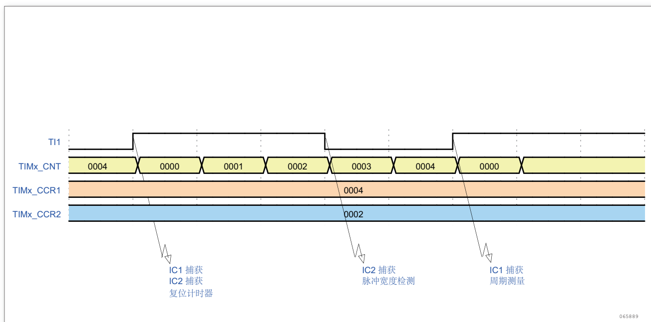
图 112. PWM 输入模式时序
