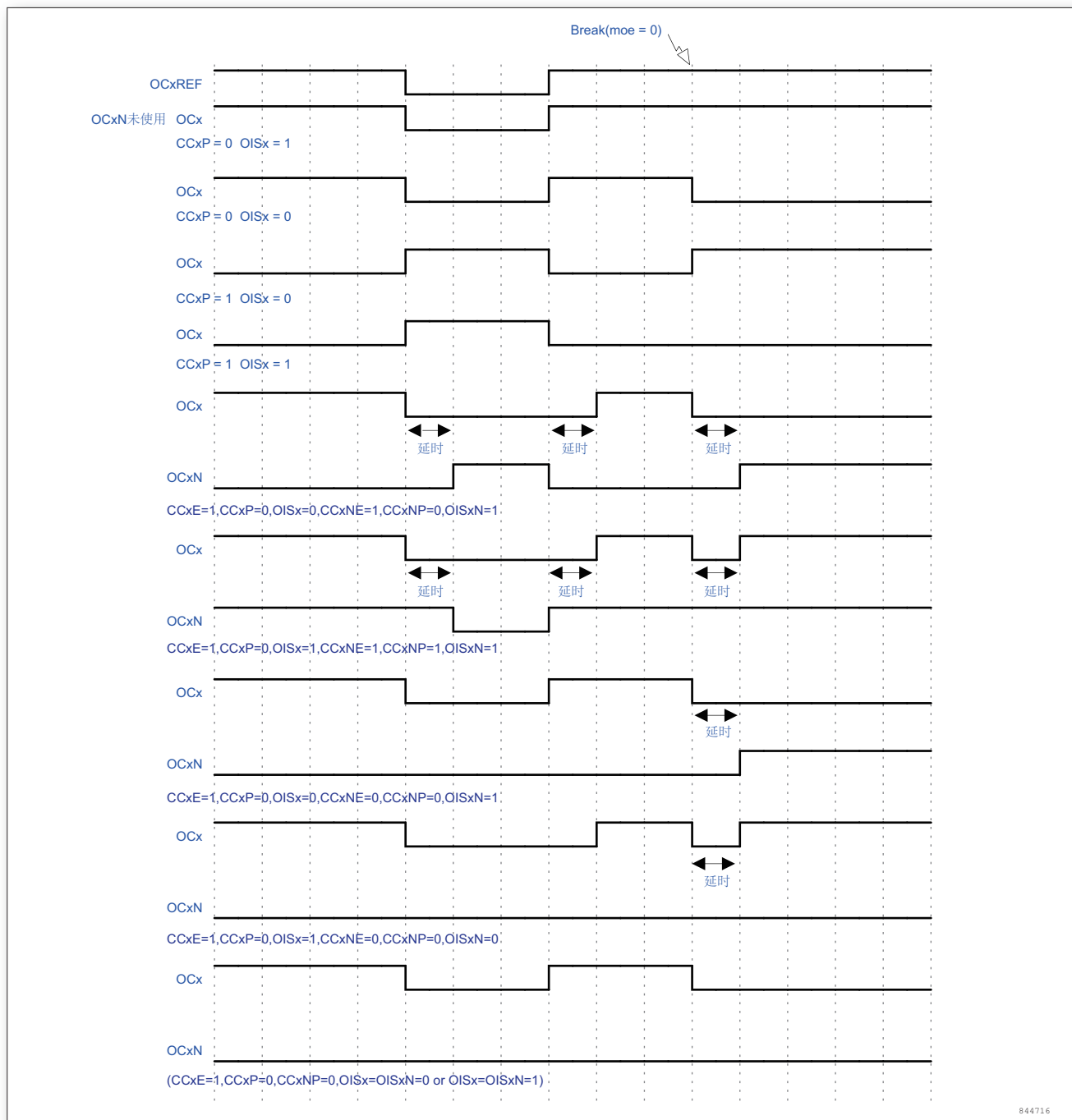
图 73. 响应刹车的输出
