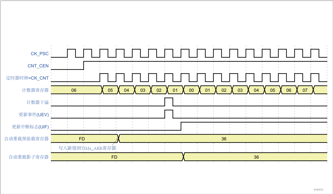
图 123. 外部时钟模式 2 + 触发模式下的控制电路
