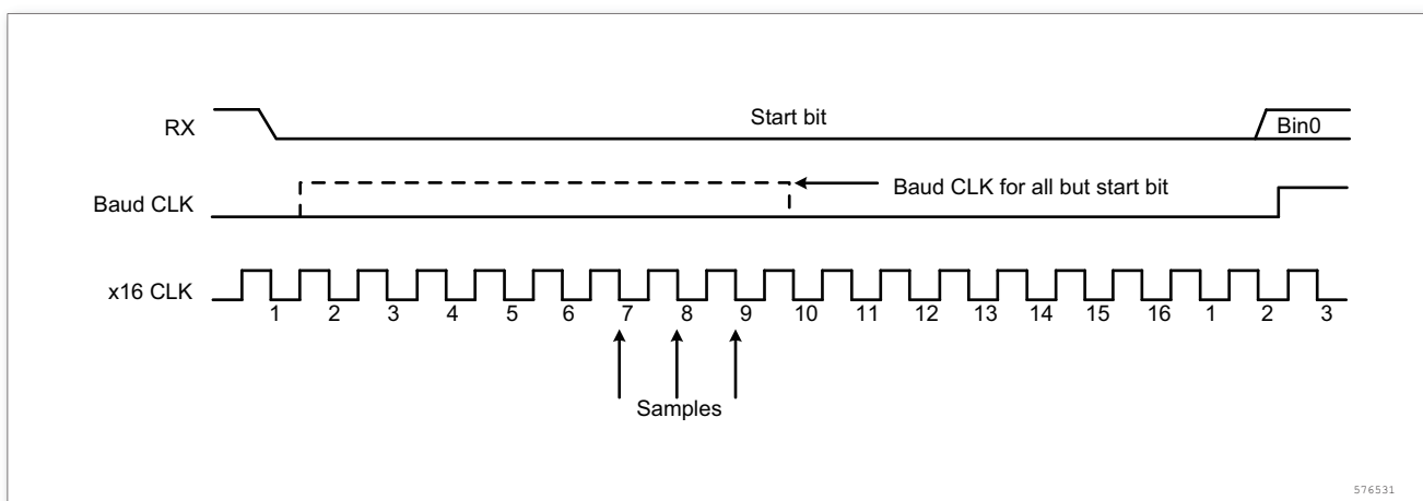
图 175. RX 引脚采样方案
