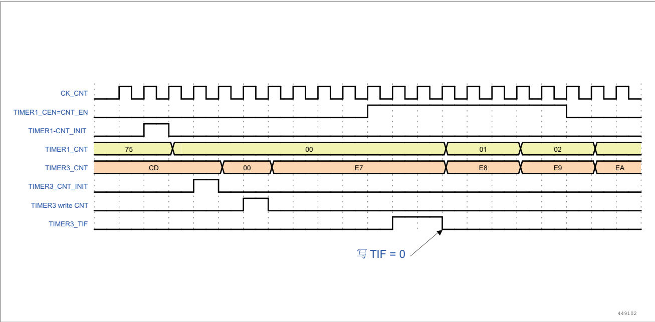
图 128. 利用定时器 1 的使能触发定时器 2
