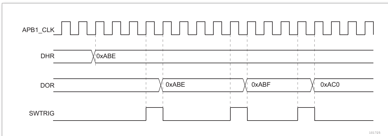
图 35. 带三角生成的 DAC 转换 (使能软件触发)
