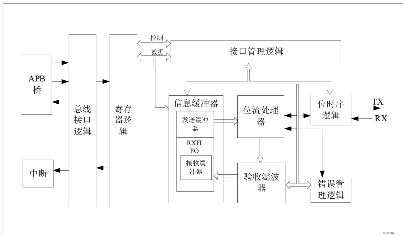
图 143. CAN 结构方框图
