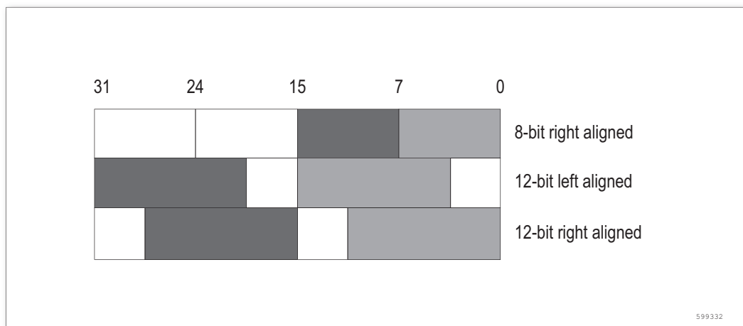
图 30. 双 DAC 通道模式的数据寄存器
