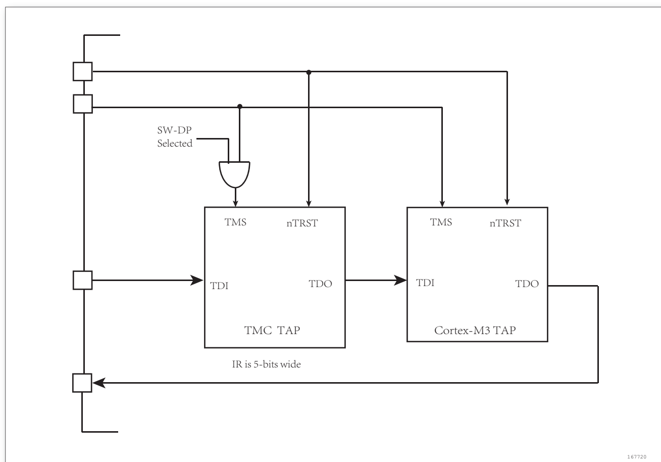
图 181. JTAG TAP 连接
