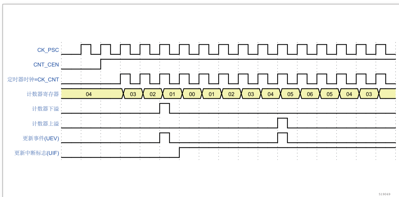
图 50. 计数器时序图，内部时钟分频因子为 1，TIMx_ARR = 0x06
