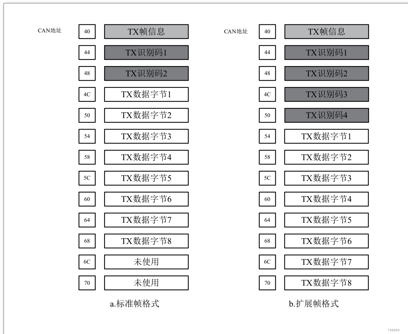
图 149. 标准帧和扩展帧格式配置在发送缓冲器的列表
