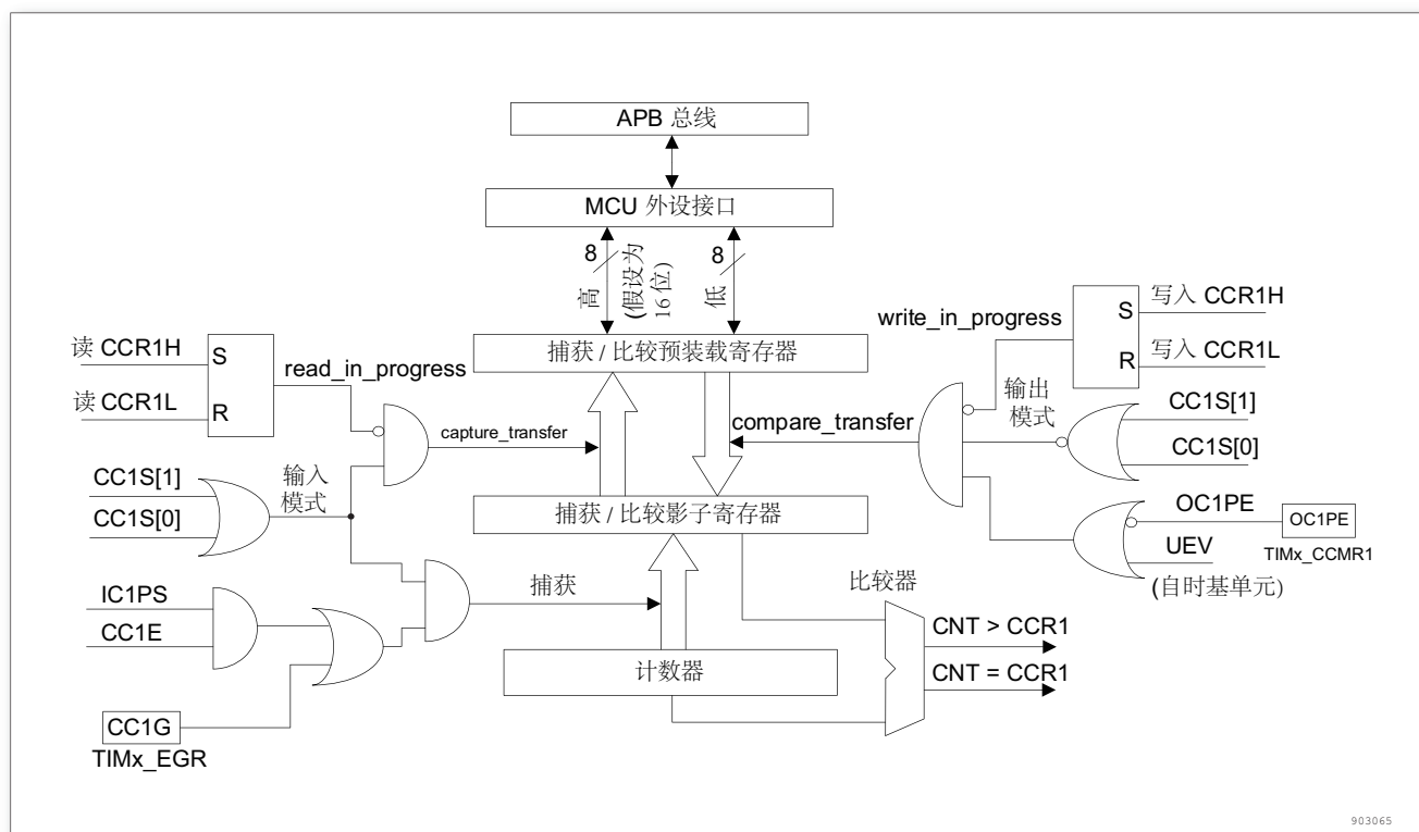
图 110. 捕获/比较通道 1 的主电路
