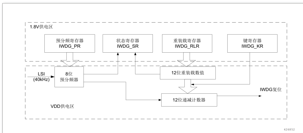
图 133. 独立看门狗框图
