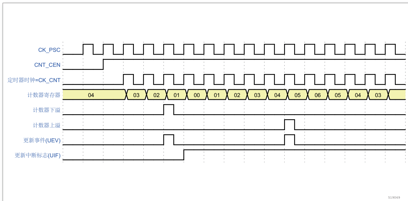
图 98. 计数器时序图，内部时钟分频因子为 1，TIMx_ARR = 0x06
