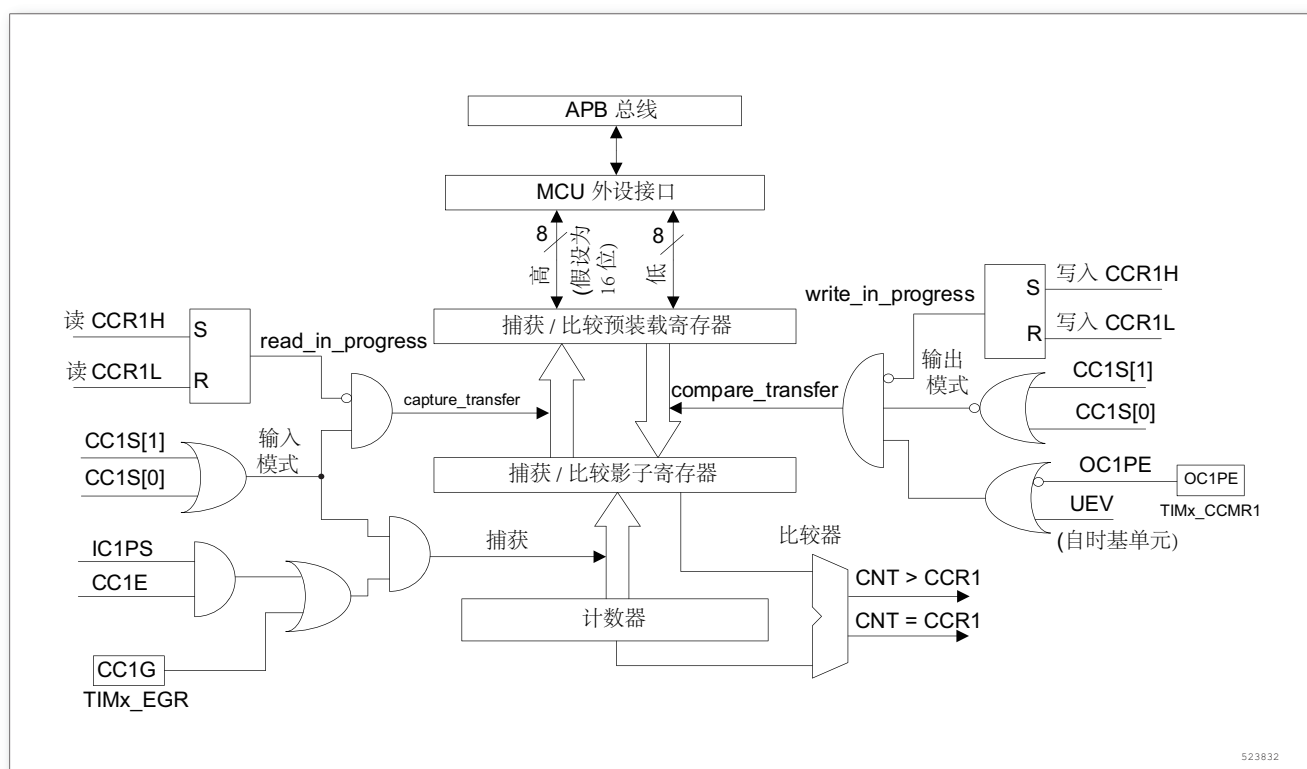
图 63. 捕获/比较通道 1 的主电路
