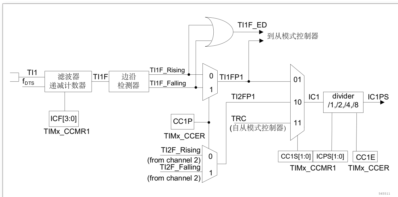
图 109. 捕获/比较通道 (如: 通道 1 输入部分)
