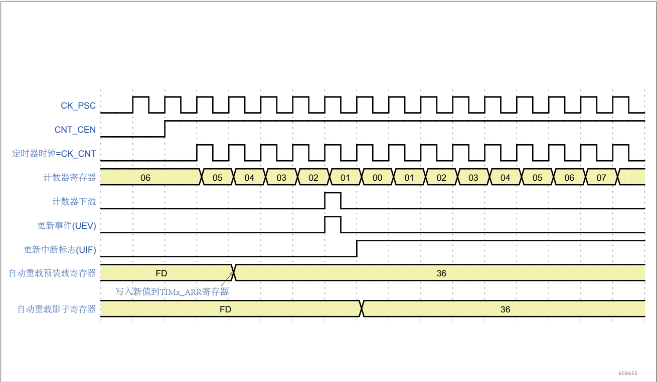
图 102. 计数器时序图，ARPE = 1 时的更新事件 (计数器下溢)
