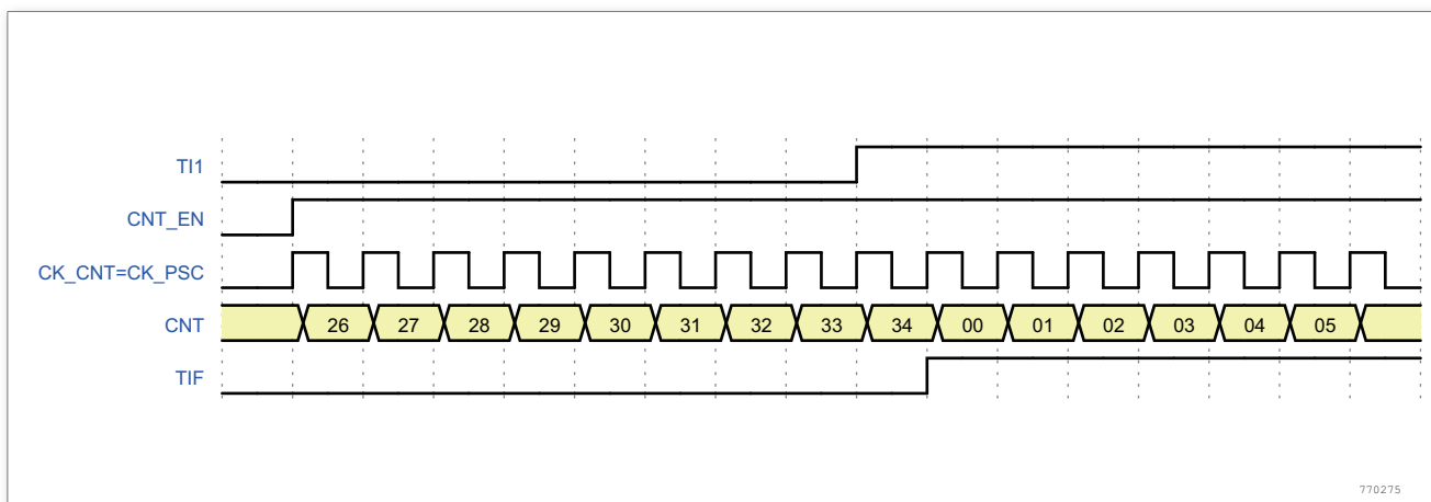
图 120. 复位模式下的控制电路
