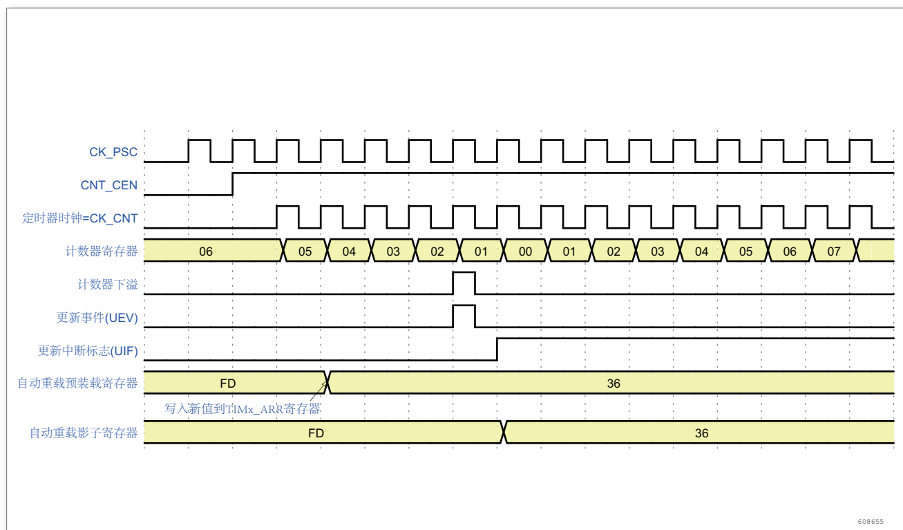
图 54. 计数器时序图，ARPE = 1 时的更新事件 (计数器下溢)
