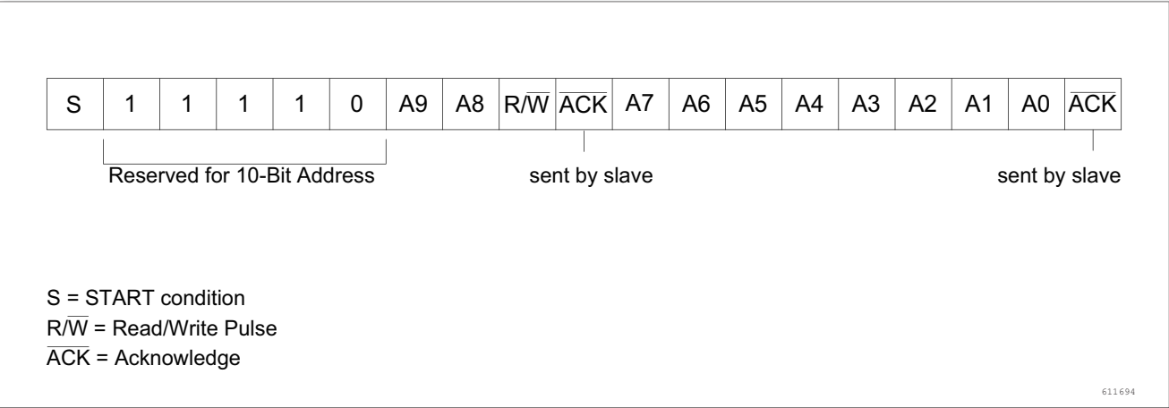
图 158. 10 位的地址格式
