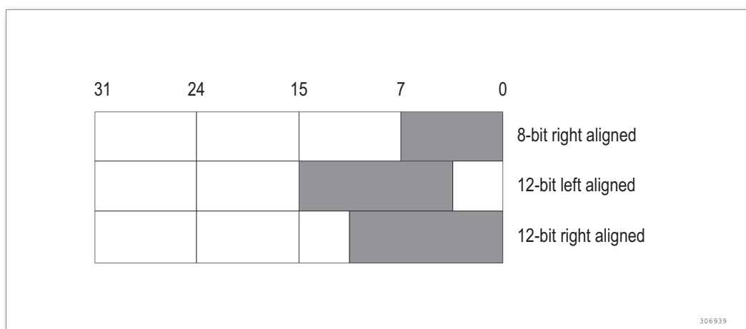
图 29. 单 DAC 通道模式的数据寄存器
