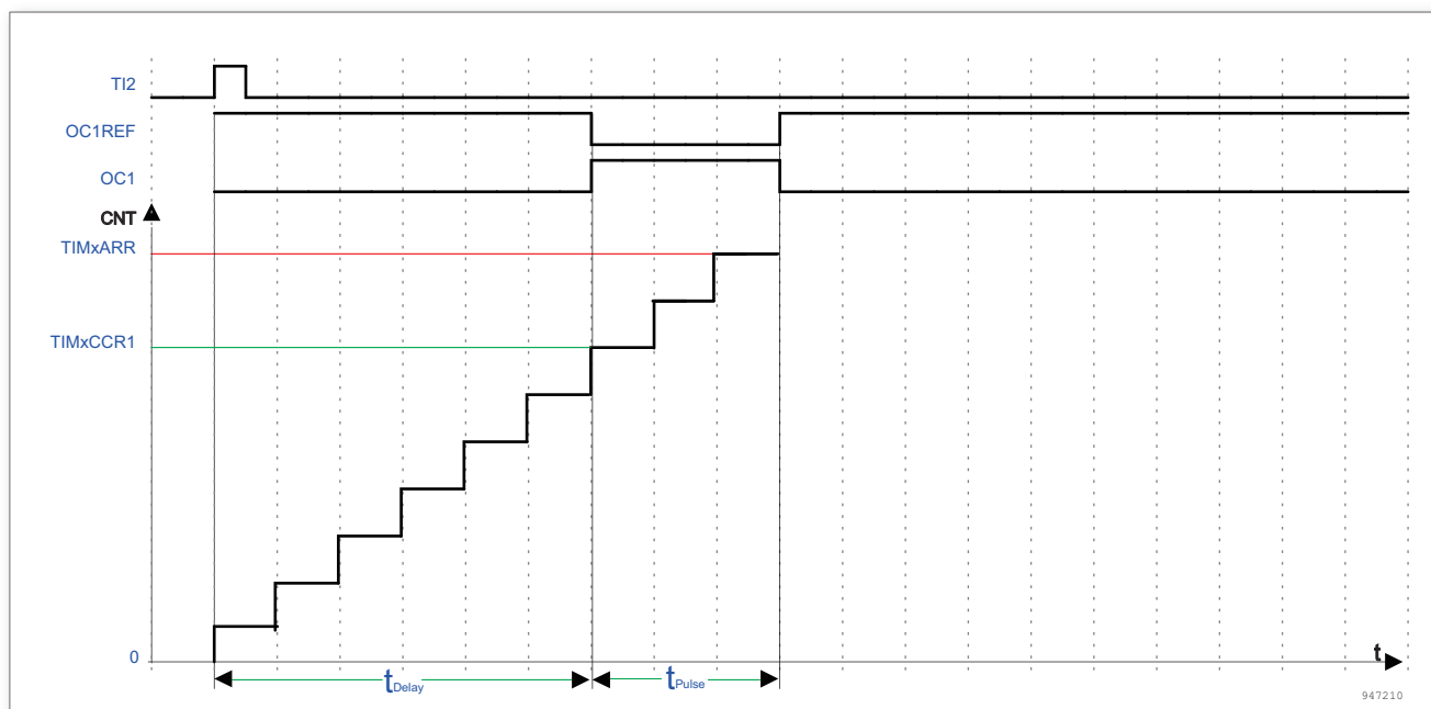
图 76. 单脉冲模式的例子
