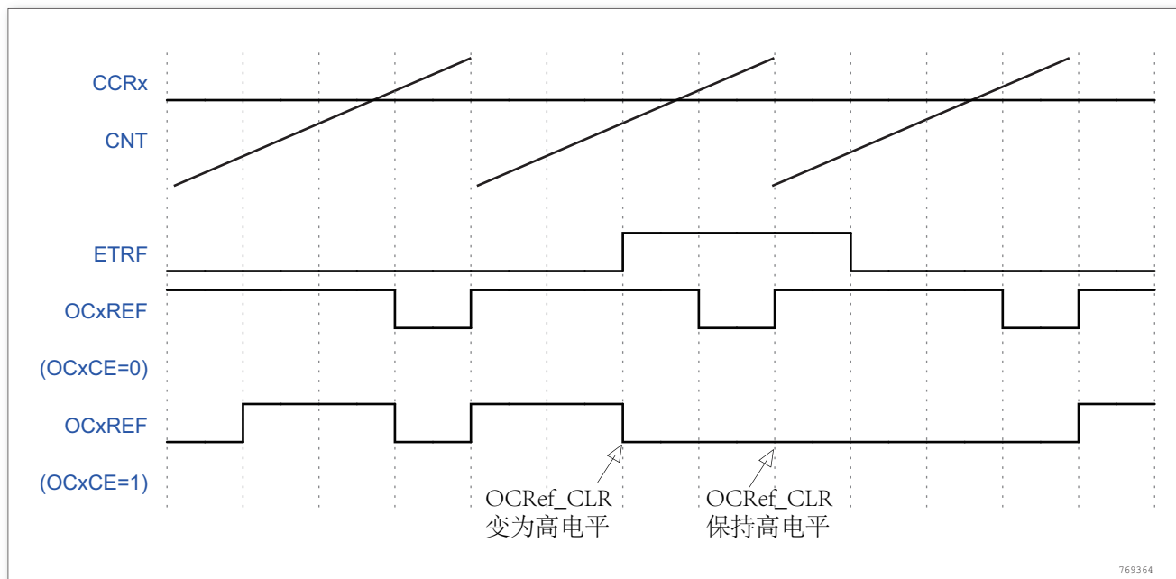
图 74. 清除 TIMx 的 OCxREF
