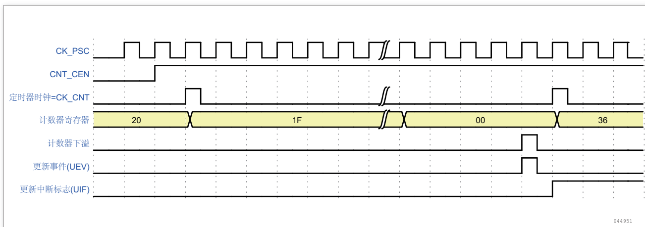
图 48. 计数器时序图, 内部时钟分频因子为 N
