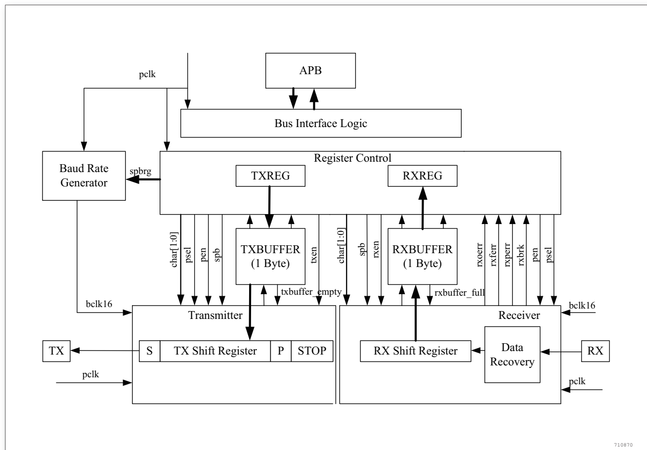
图 170. UART 方框图
