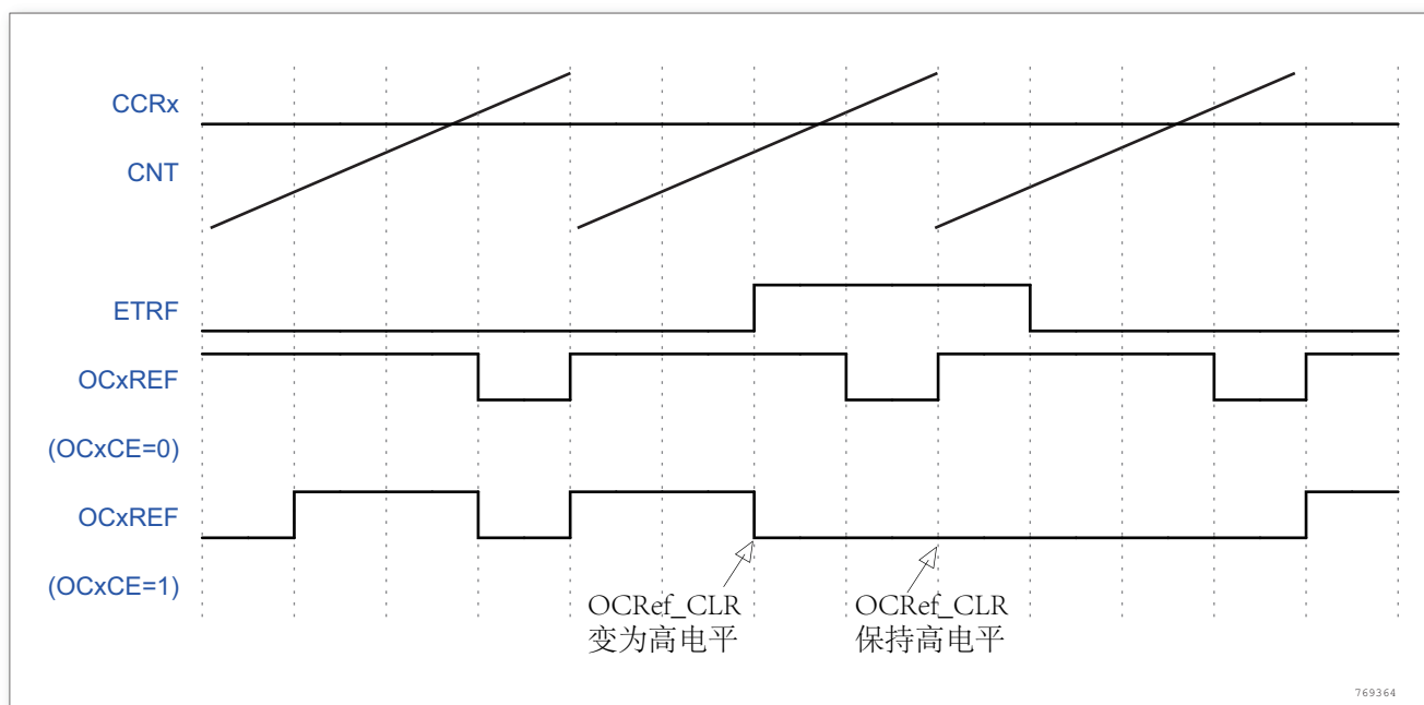
图 117. 清除 TIMx 的 OCxREF
