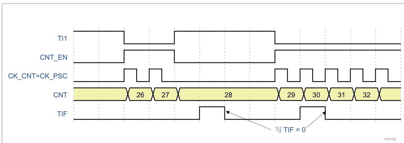
图 81. 门控模式下的控制电路
