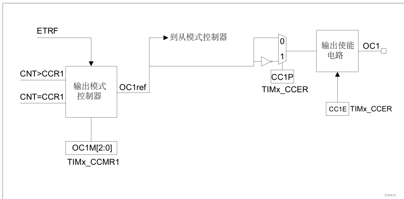
图 111. 捕获/比较通道的输出部分 (通道 1)
