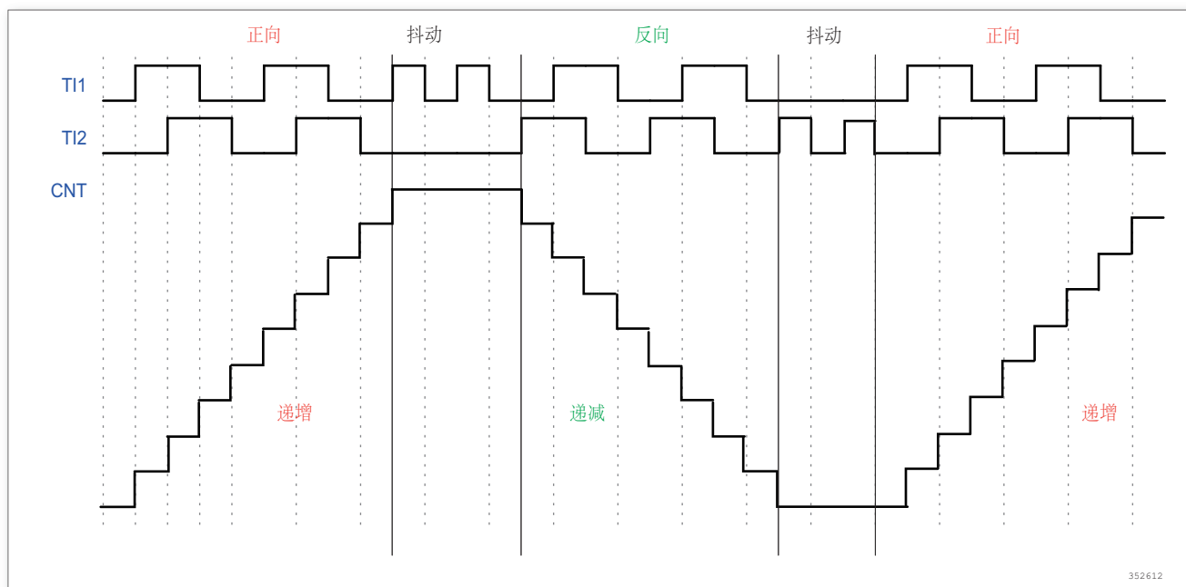
图 118. 编码器模式下的计数器操作实例
