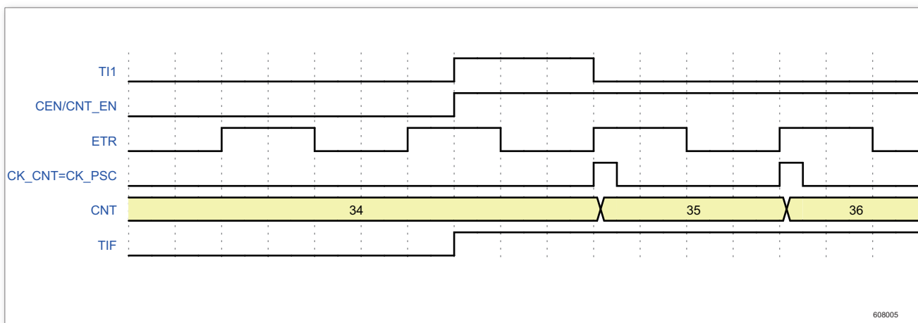
图 83. 外部时钟模式 2 + 触发模式下的控制电路
