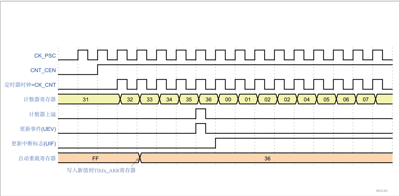
图 91. 计数器时序图，当 ARPE = 0 时的更新事件 (TIMx_ARR 没有预装入)
