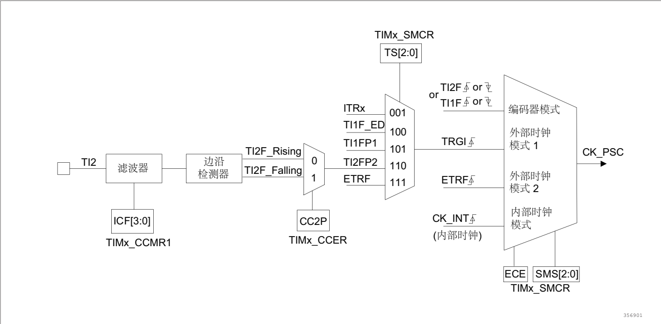
图 105. TI2 外部时钟连接例子
