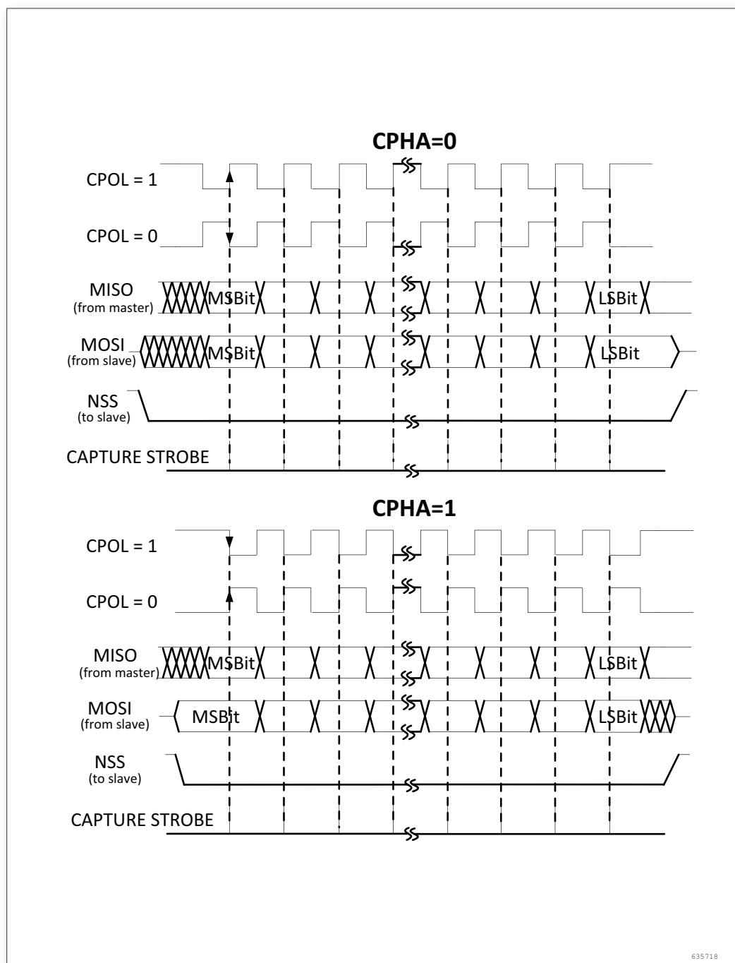
图 155. 数据时钟时序图
