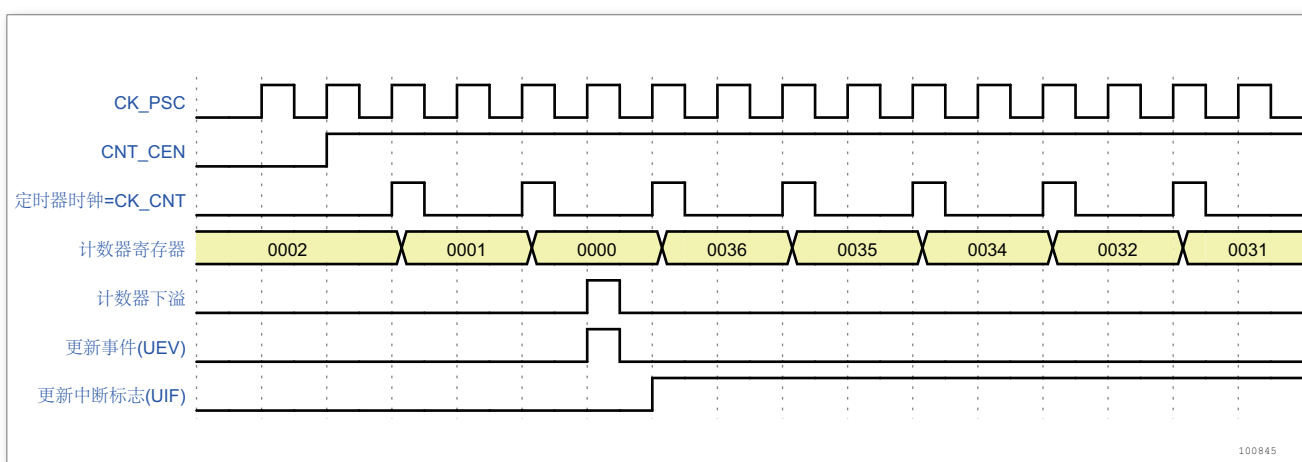
图 94. 计数器时序图，内部时钟分频因子为 2
