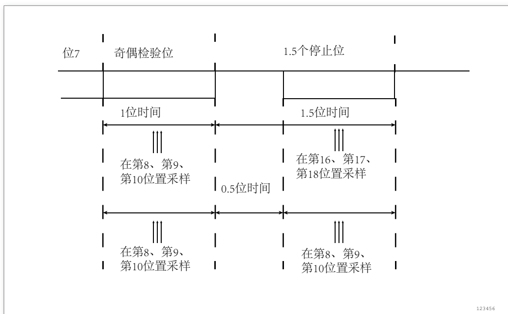
图 174. UART 方框图
