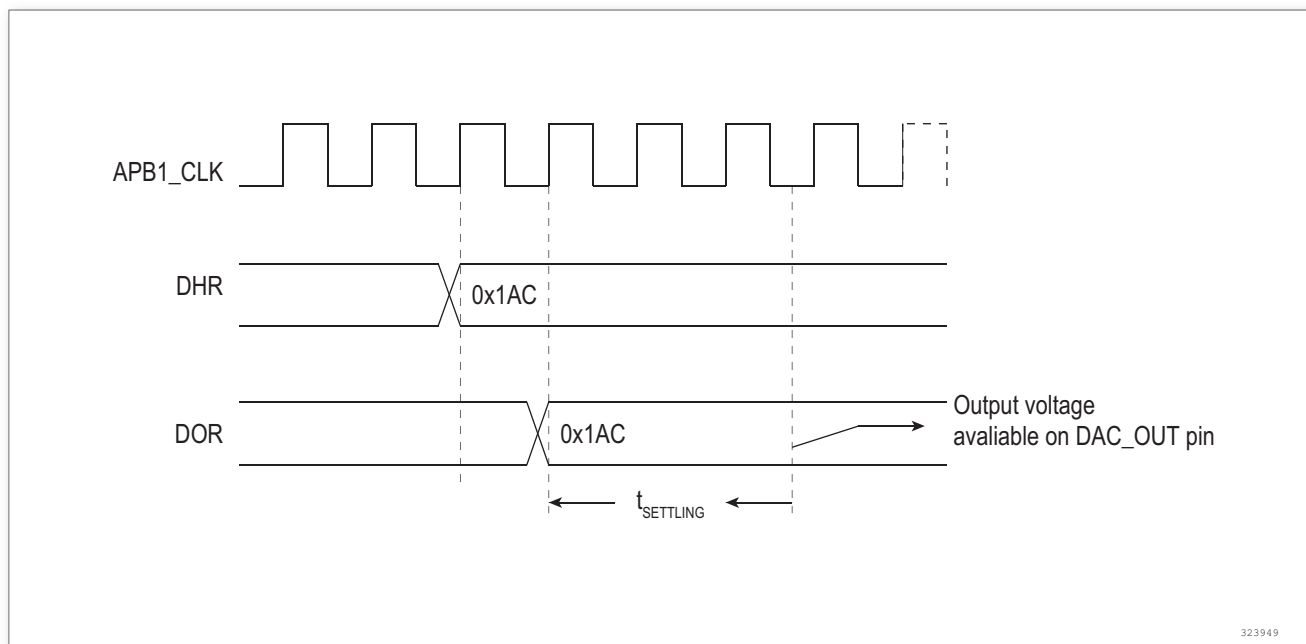
图 31. TEN = 0 触发关闭时转换的时间框图
