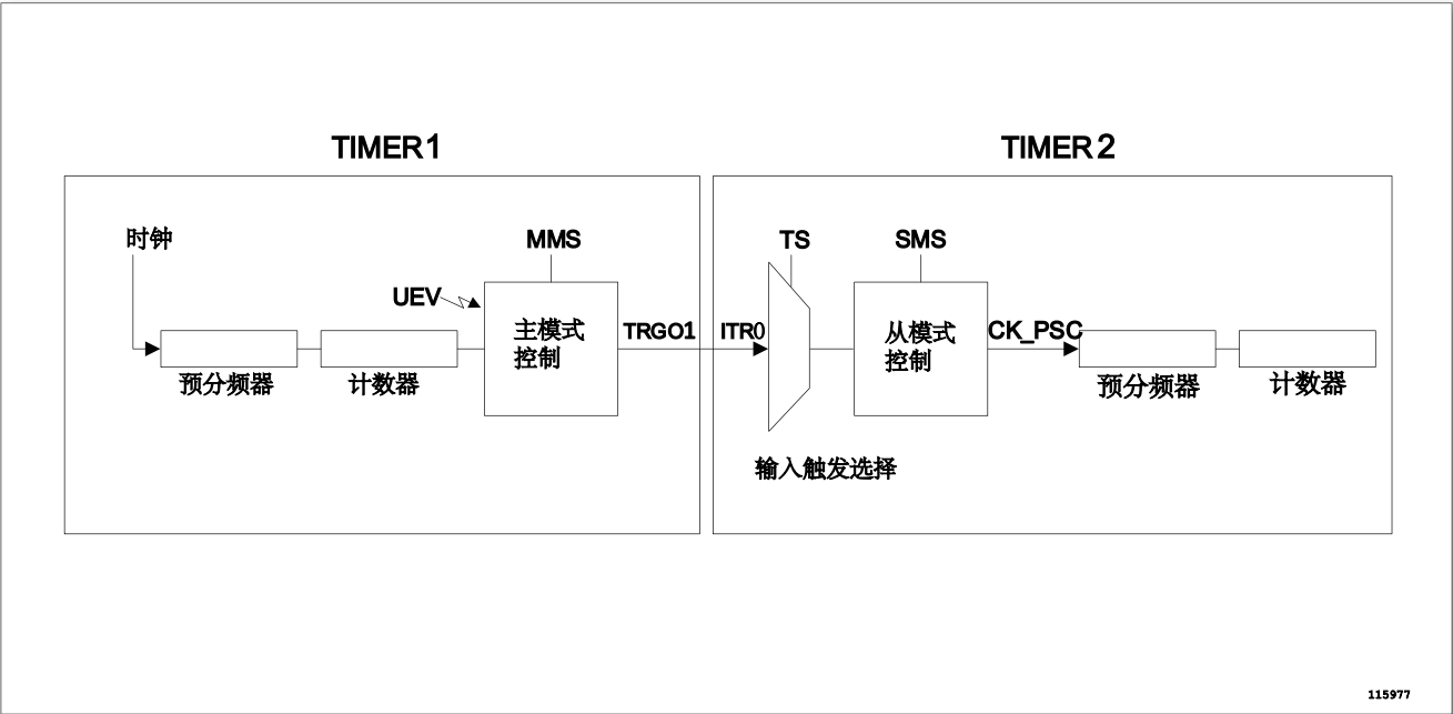
图 124. 主/从定时器的例子
