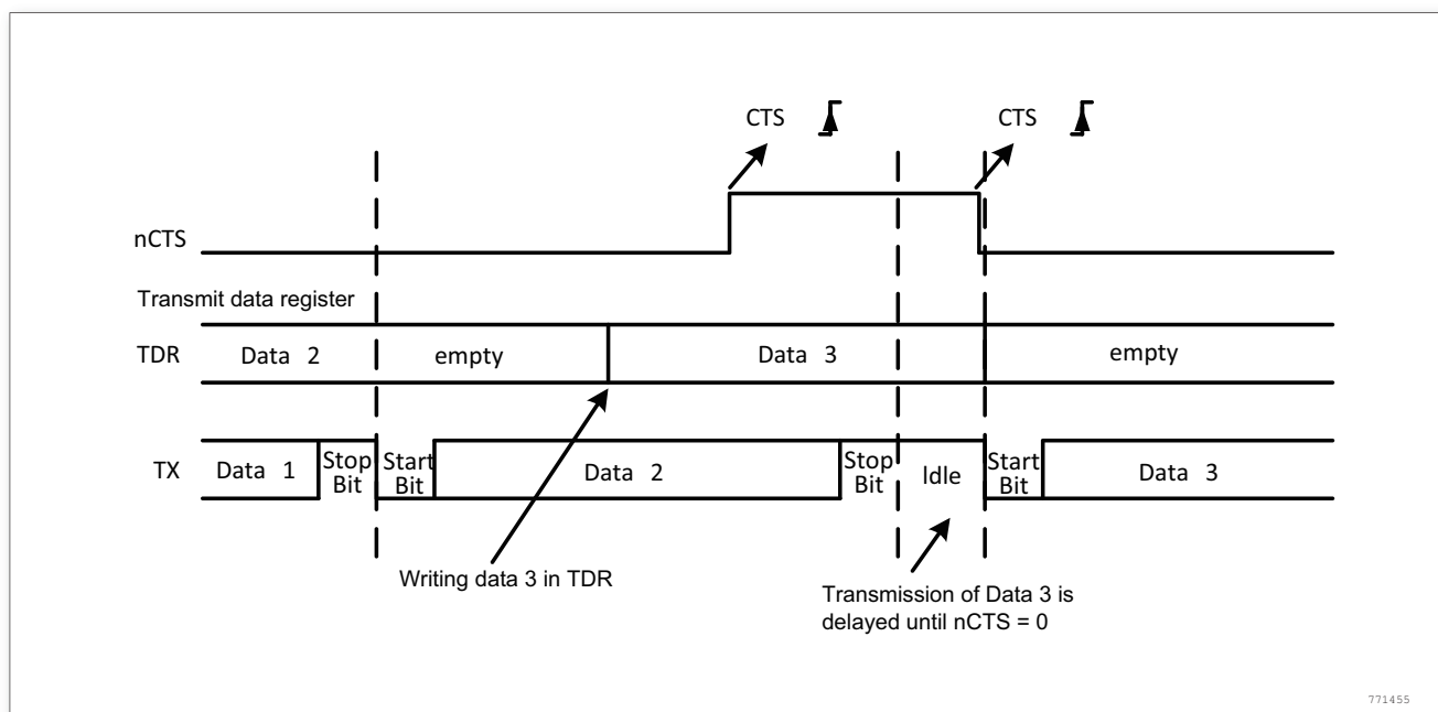
图 178. CTS 流控制
