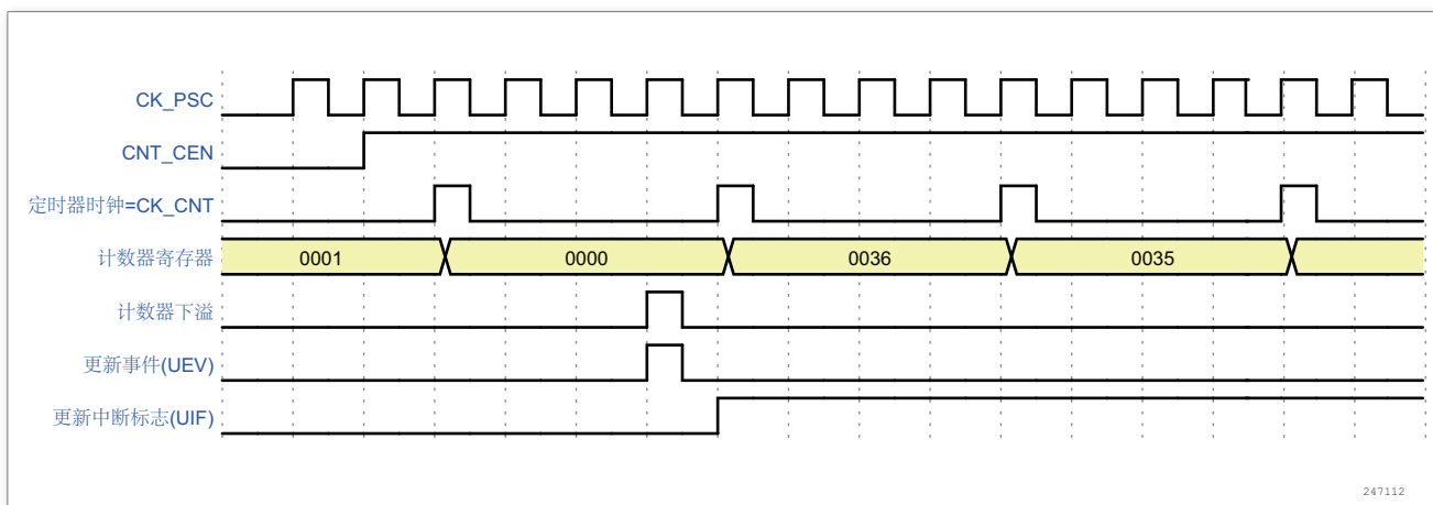
图 95. 计数器时序图，内部时钟分频因子为 4
