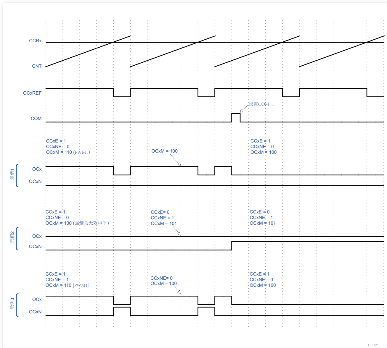
图 75. 产生六步 PWM，使用 COM 的例子 (OSSR = 1)
