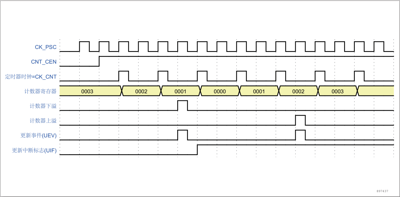
图 51. 计数器时序图，内部时钟分频因子为 2
