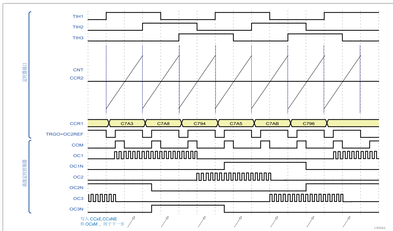
图 79. 霍尔传感器接口的实例
