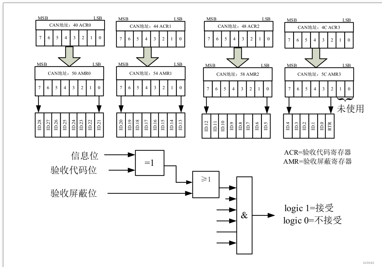
图 146. 单滤波器配置，接收扩展帧信息
