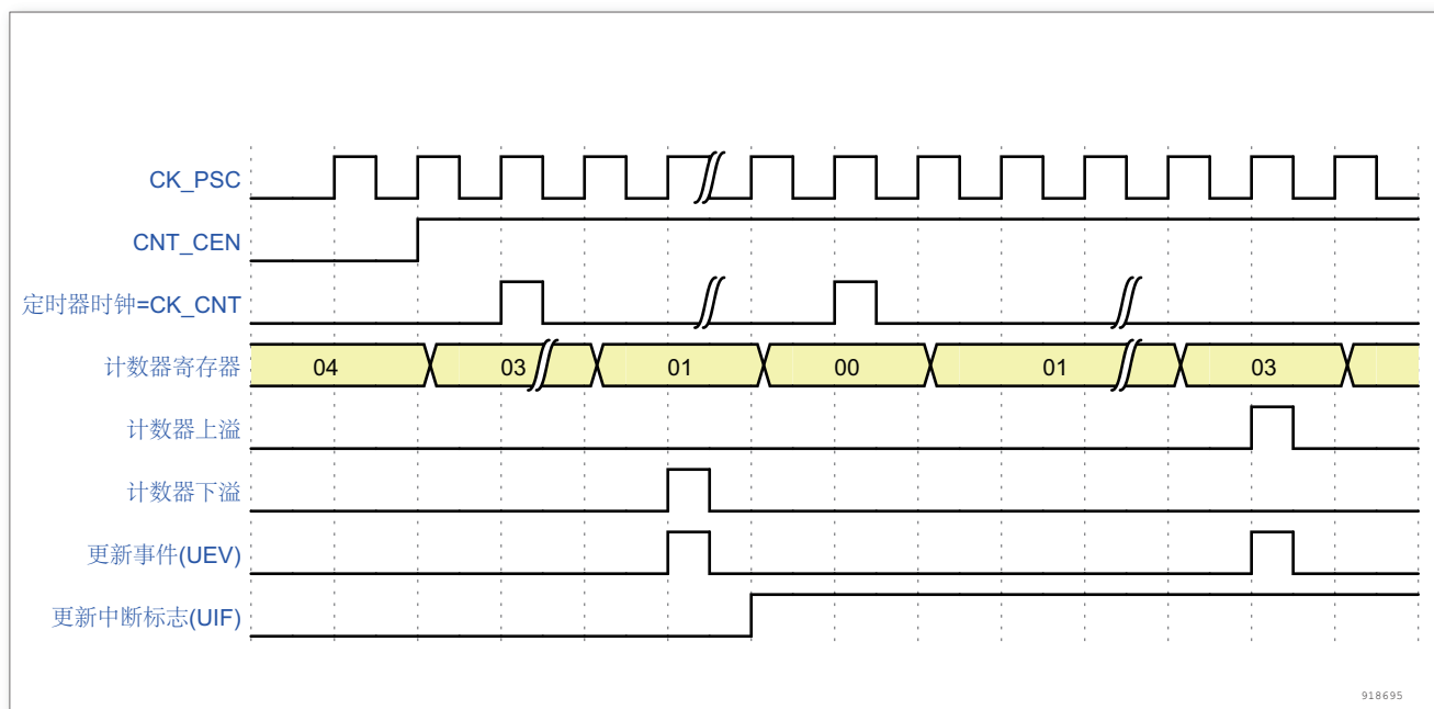
图 53. 计数器时序图，内部时钟分频因子为 N
