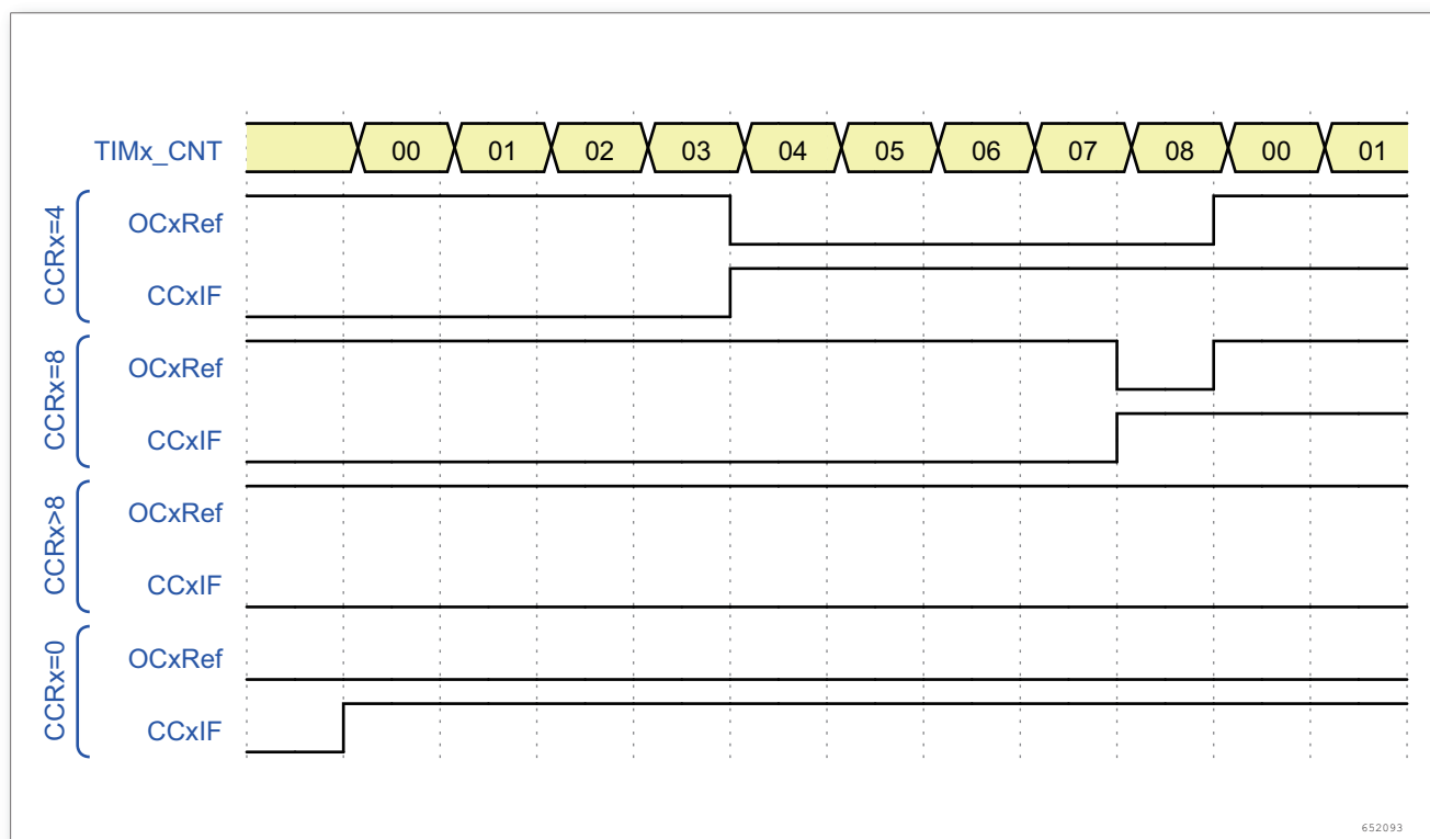
图 68. 边沿对齐的 PWM 波形 (ARR = 8)
