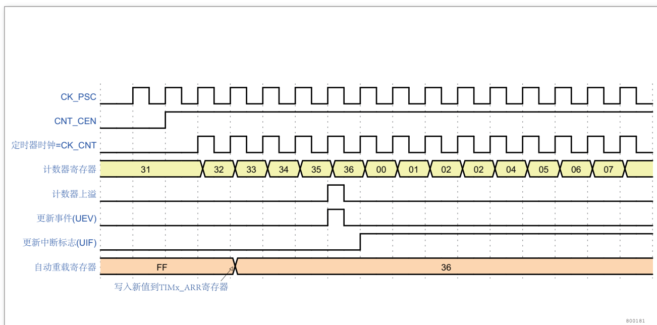
图 43. 计数器时序图, 当 ARPE = 0 时的更新事件 (TIMx_ARR 没有预装入)
