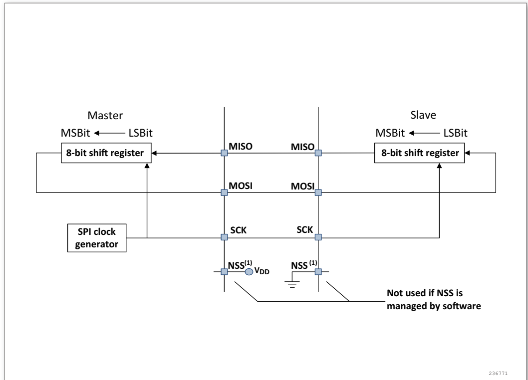
图 154. 单主和单从应用
