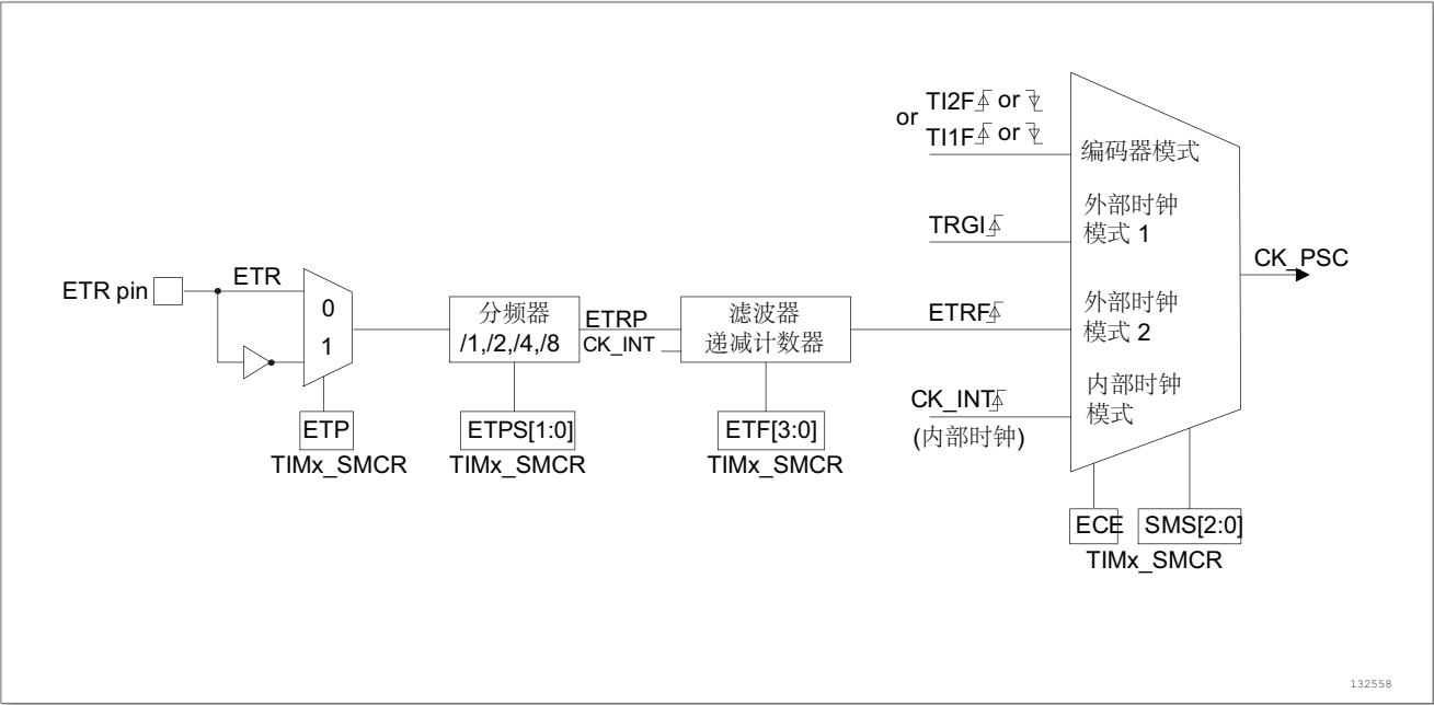
图 107. 外部触发输入框图
