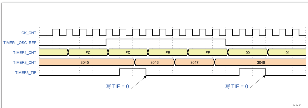
图 125. 定时器 1 的 OC1REF 控制定时器 2
