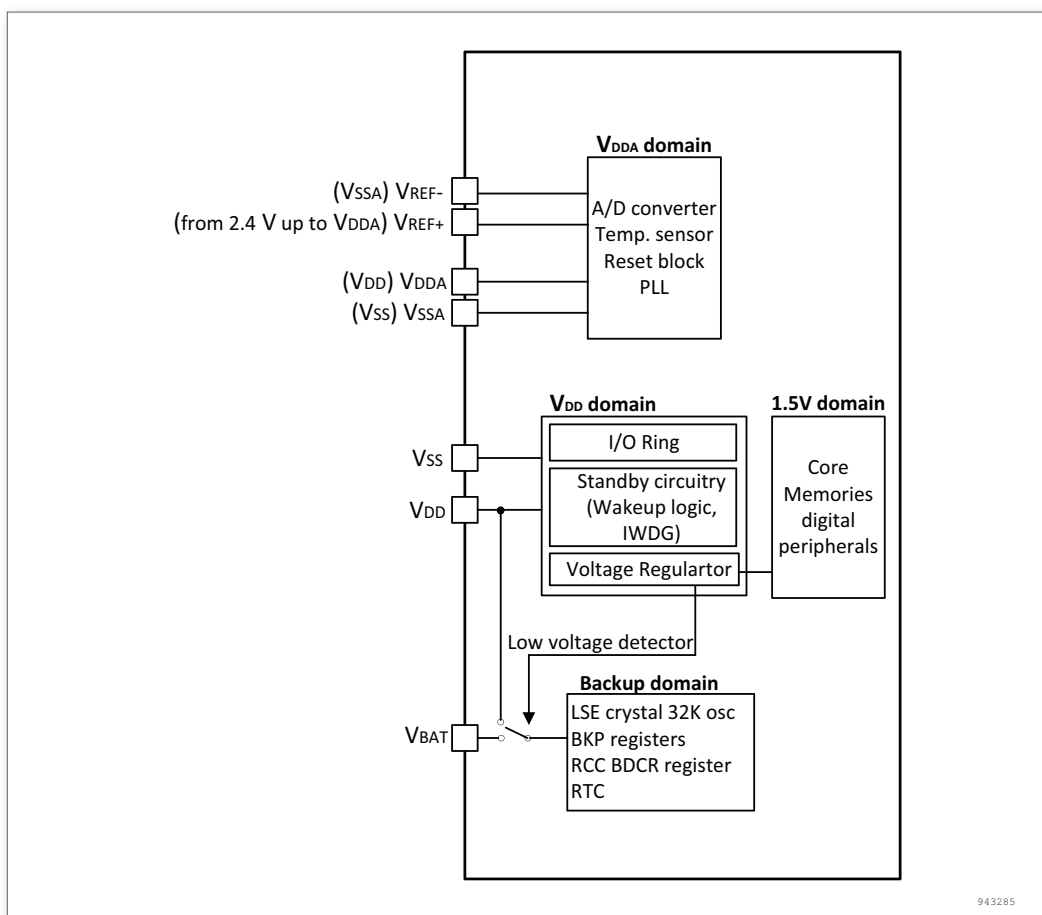
图 8. 电源框图
