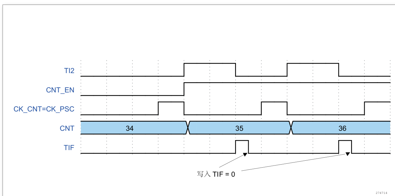
图 106. 外部时钟模式 1 下的控制电路
