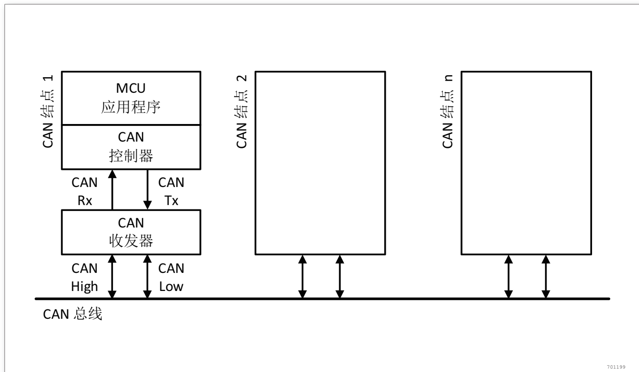
图 142. CAN 网络拓扑结构
