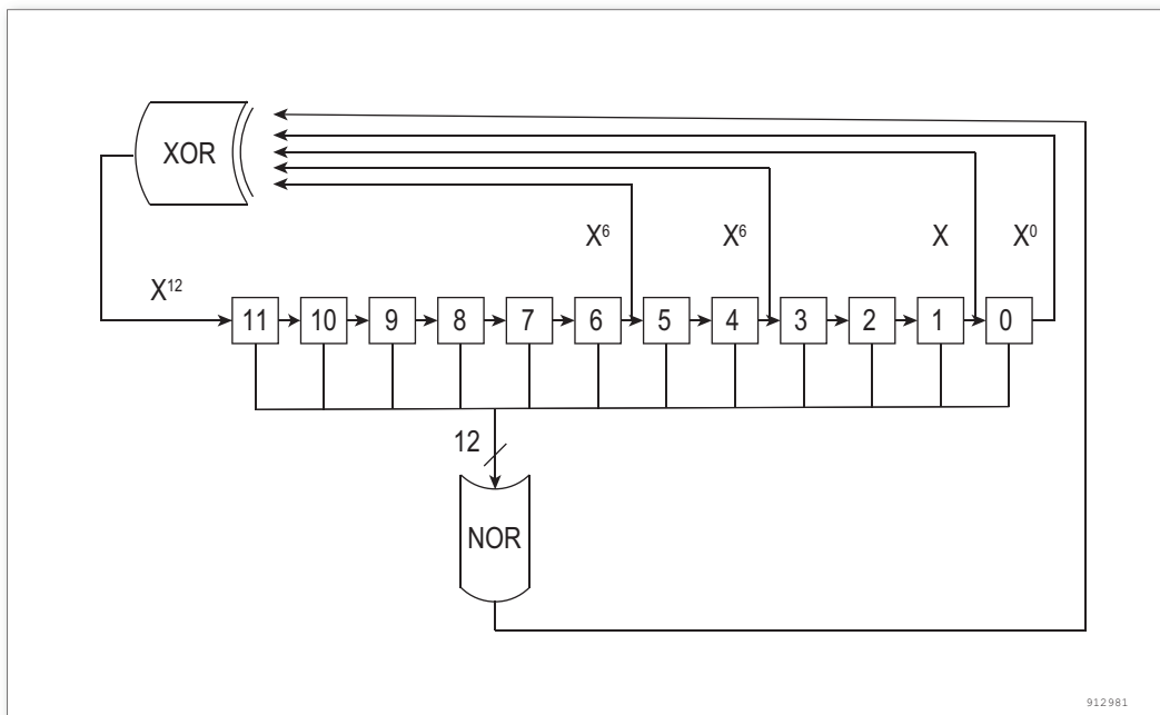
图 32. DAC LFSR 寄存器算法
